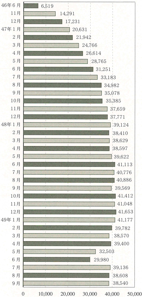
グラフ1 軍作業員数の推移 (41)
