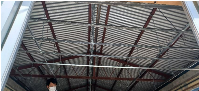
天井軽鉄骨組
