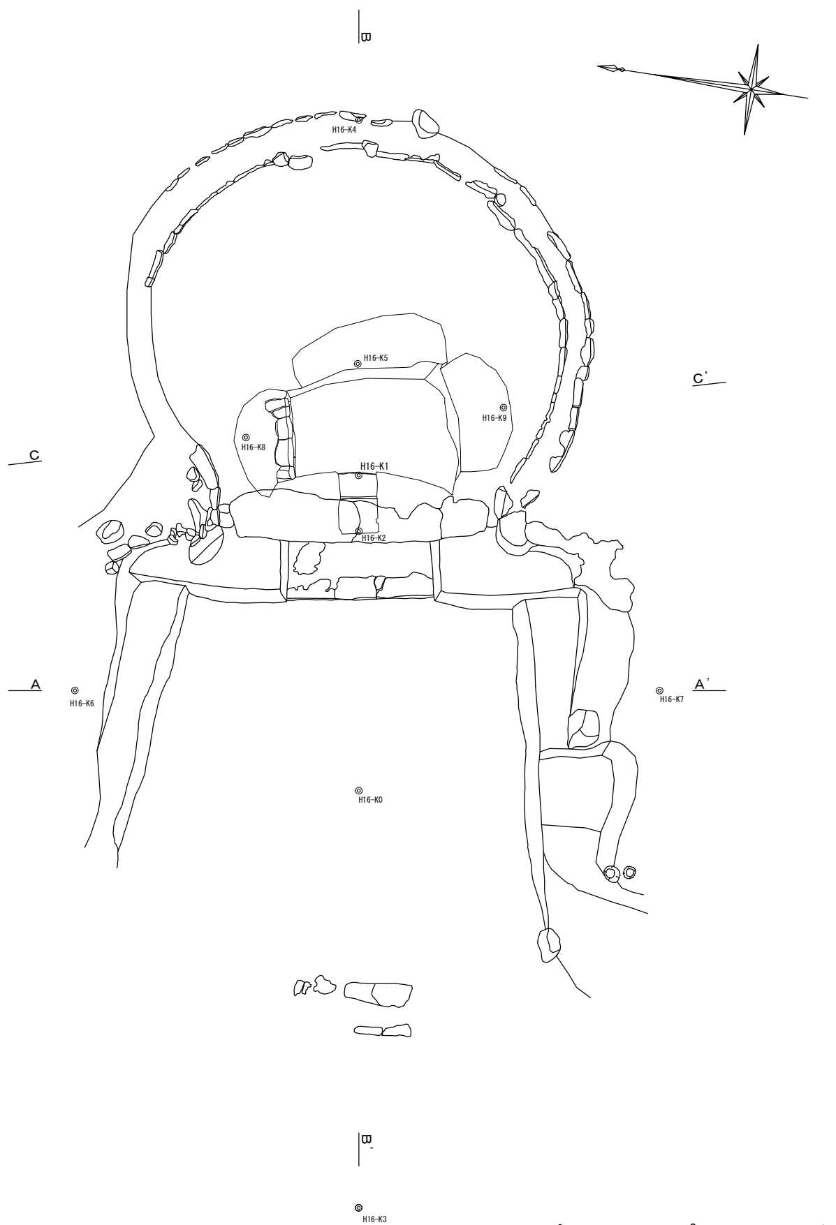
第 41 图 016号墓 平面图
