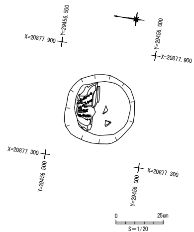
第 72 図 墓庭埋納蔵骨器 出土平面図
