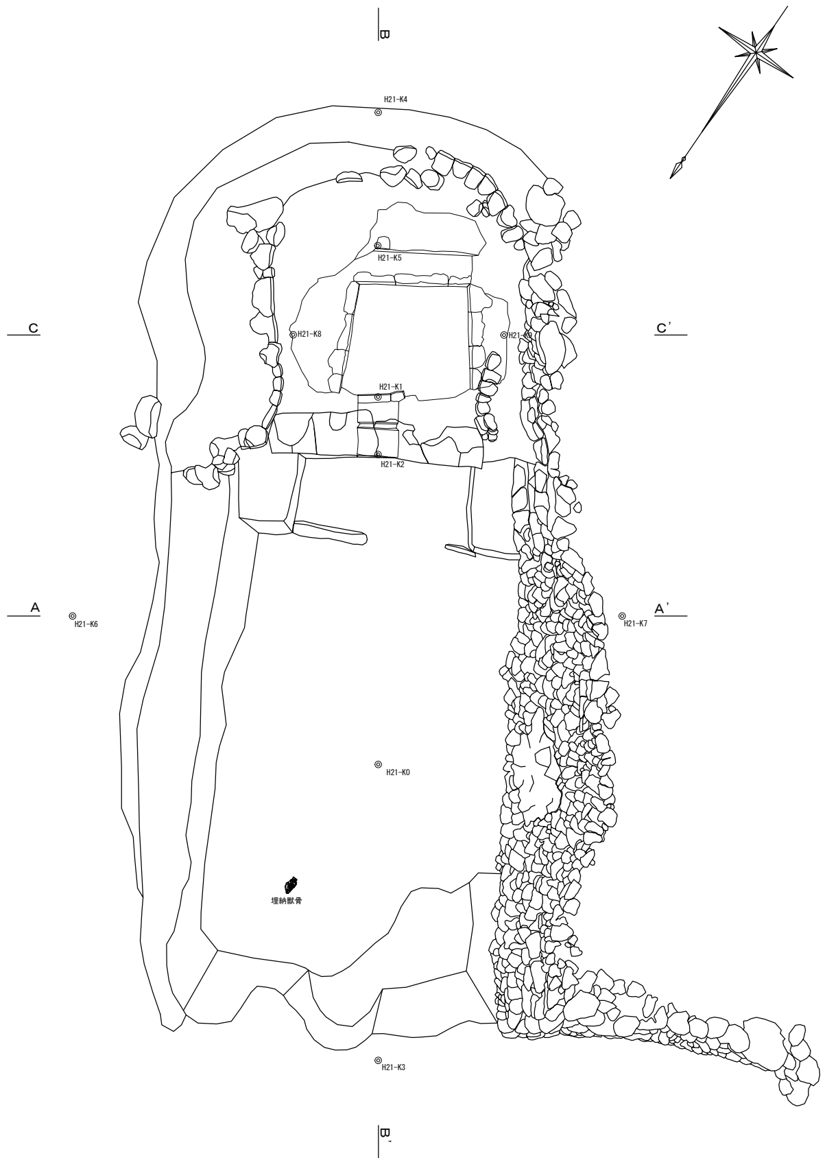
第 52 图 021号墓 平面图
