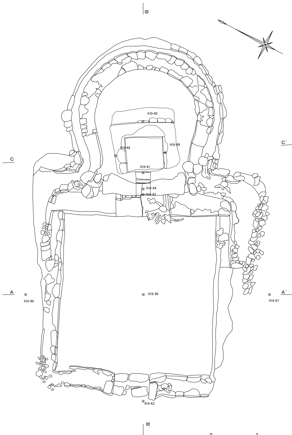
第 44 图 018号墓 平面图
