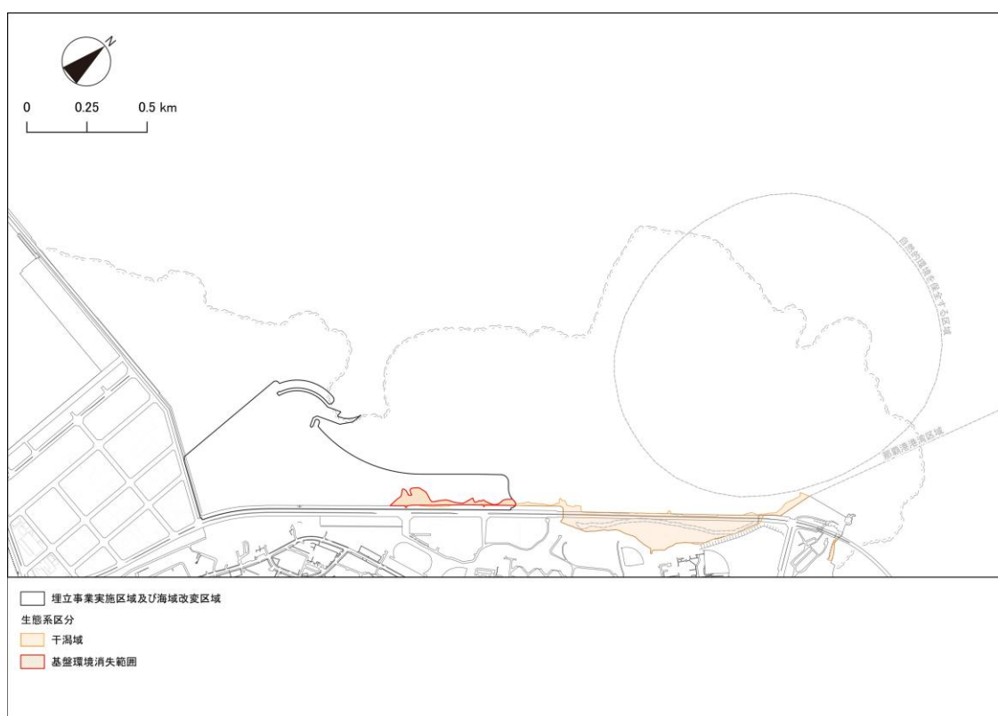
図 6.12.31 藻場域と海域改変区域の重ね合わせ（消失範囲）
