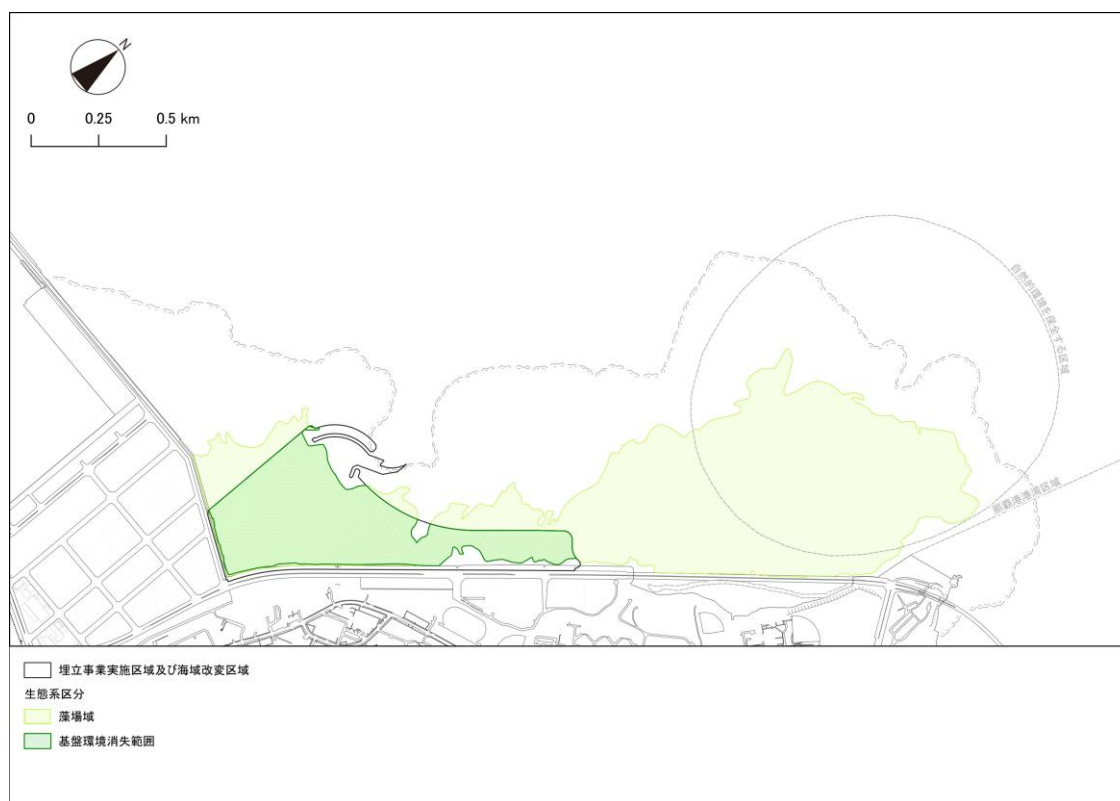
図 6.12.27 藻場域と海域改変区域の重ね合わせ（消失範囲）
