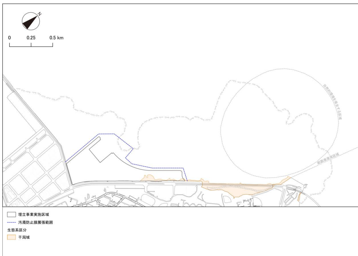
図 6.12.19 汚濁防止膜の設置範囲と干潟域の重ね合わせ
