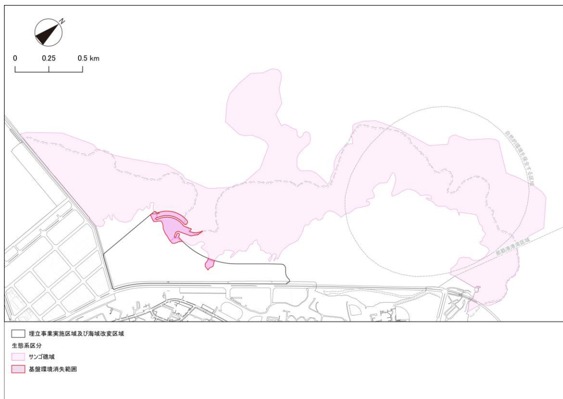
図 6.12.22 サンゴ礁域と海域改変区域の重ね合わせ（消失範囲）
