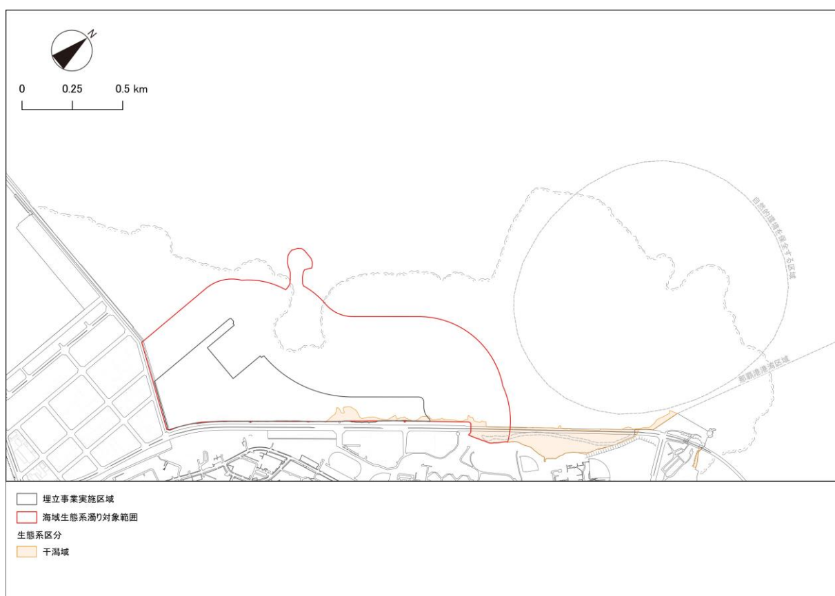
図 6.12.17 干潟域と SS 拡散範囲
