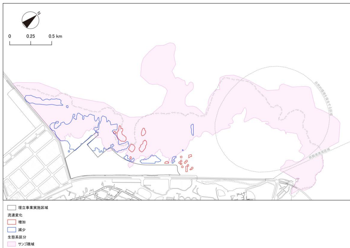
図 6.12.24 サンゴ礁域と潮流・波浪変化域
