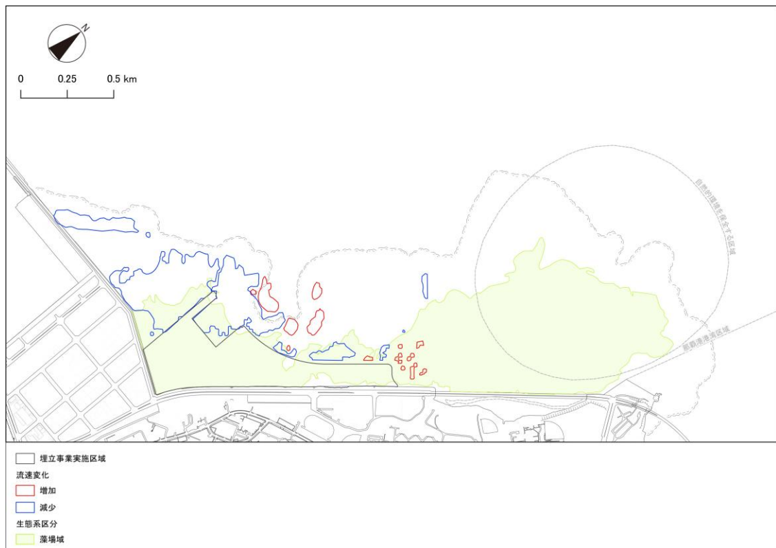
図 6.12.28 藻場域と潮流・波浪変化域の重ね合わせ
