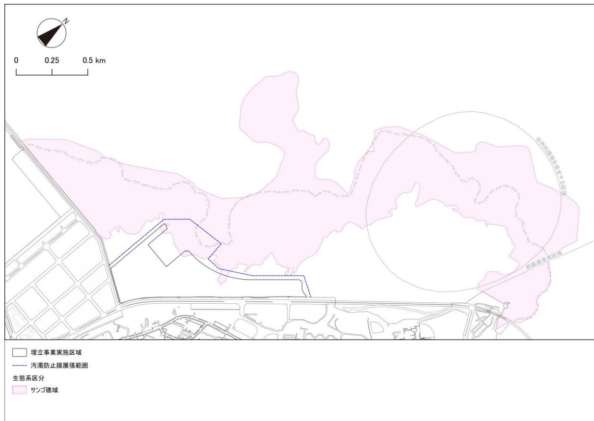
図 6.12.13 汚濁防止膜の設置範囲とサンゴ礁域の重ね合わせ
