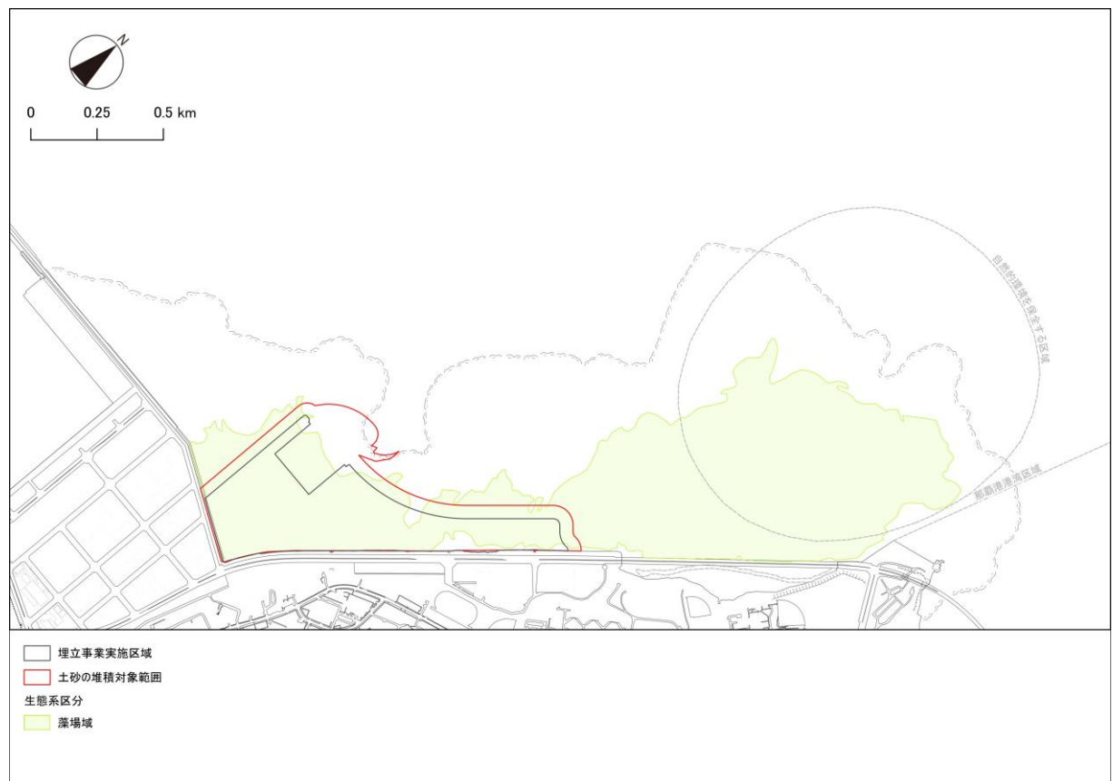
図 6.12.15 藻場域と土砂の堆積範囲
