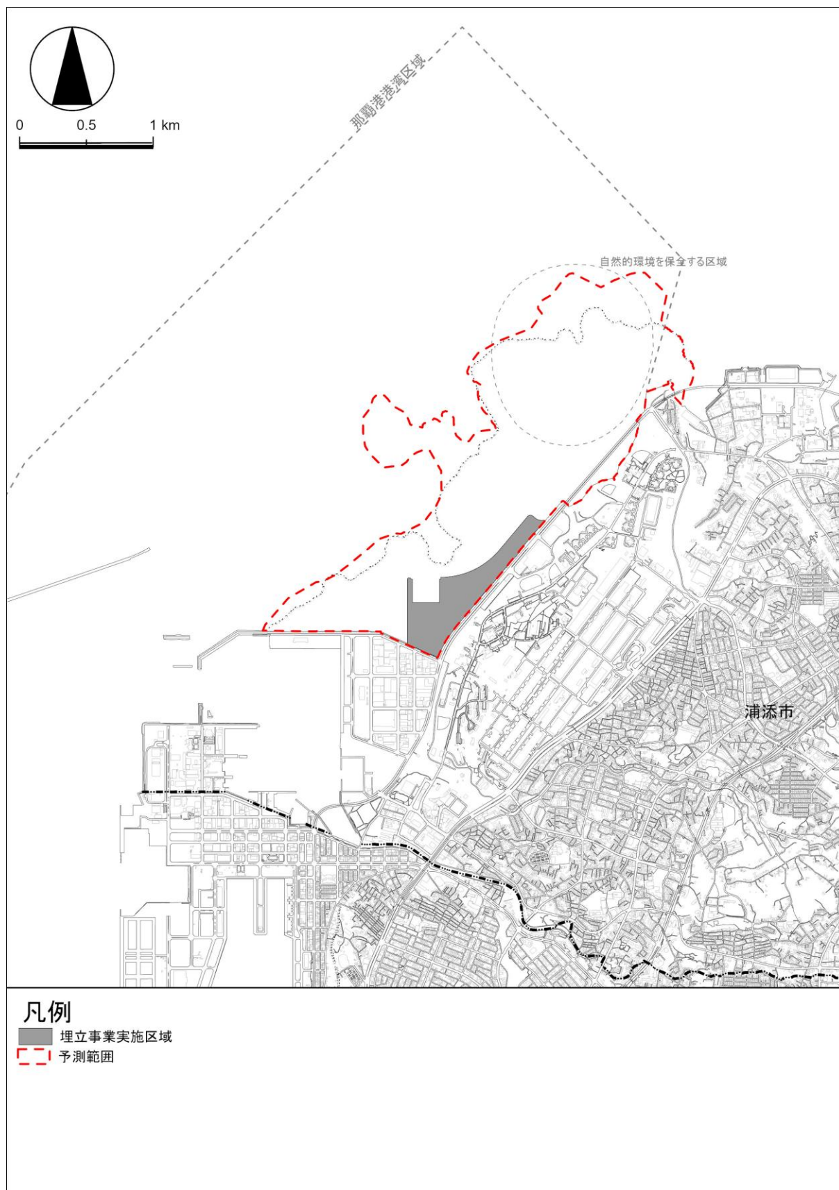
図 6.12.20 海域生態系の予測地域
