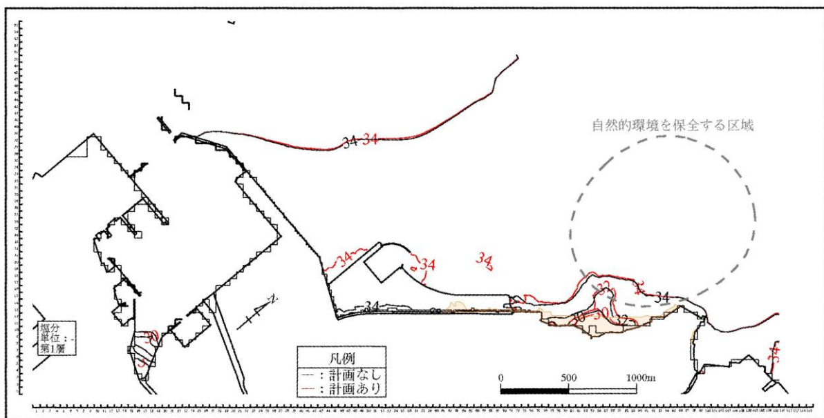
【10 年確率降雨ピーク時から 72 時間後(3 日後)、夏季】
