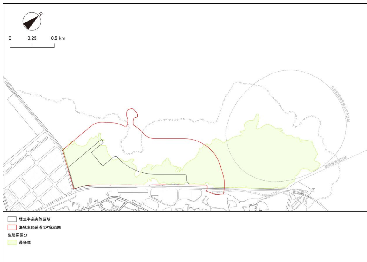
図 6.12.14 藻場域と SS 拡散範囲
