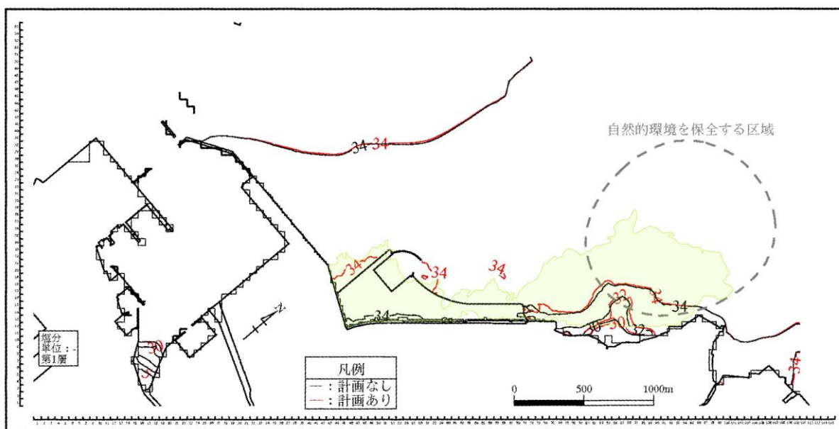
【10 年確率降雨ピーク時から 72 時間後(3 日後)、夏季】
