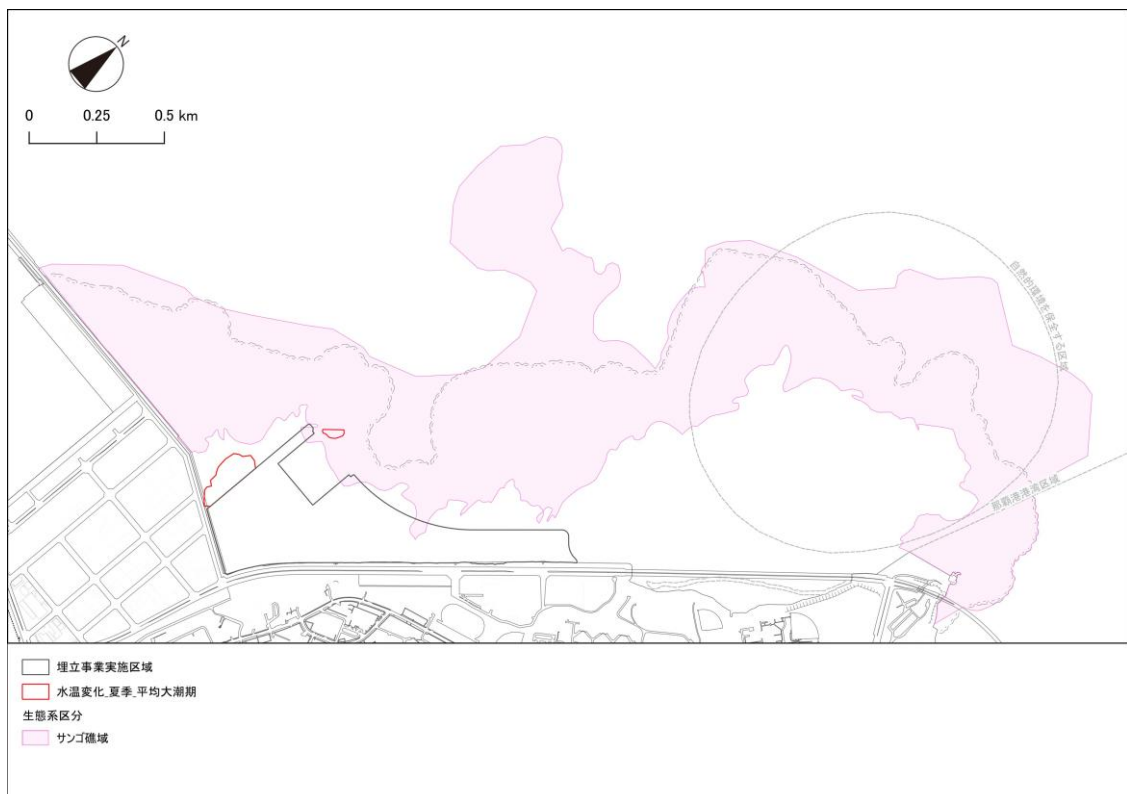
図 6.12.25 サンゴ礁域と水温予測結果（夏季）の重ね合わせ
