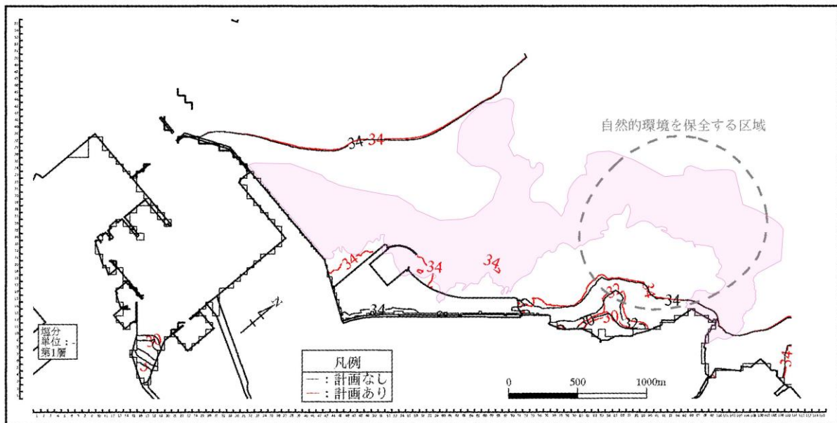
図 6.12.26 サンゴ礁域と降雨時予測結果（夏季）の重ね合わせ
