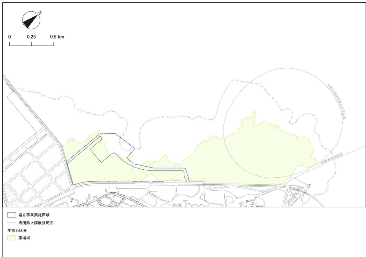
図 6.12.16 汚濁防止膜の設置範囲と藻場域の重ね合わせ
