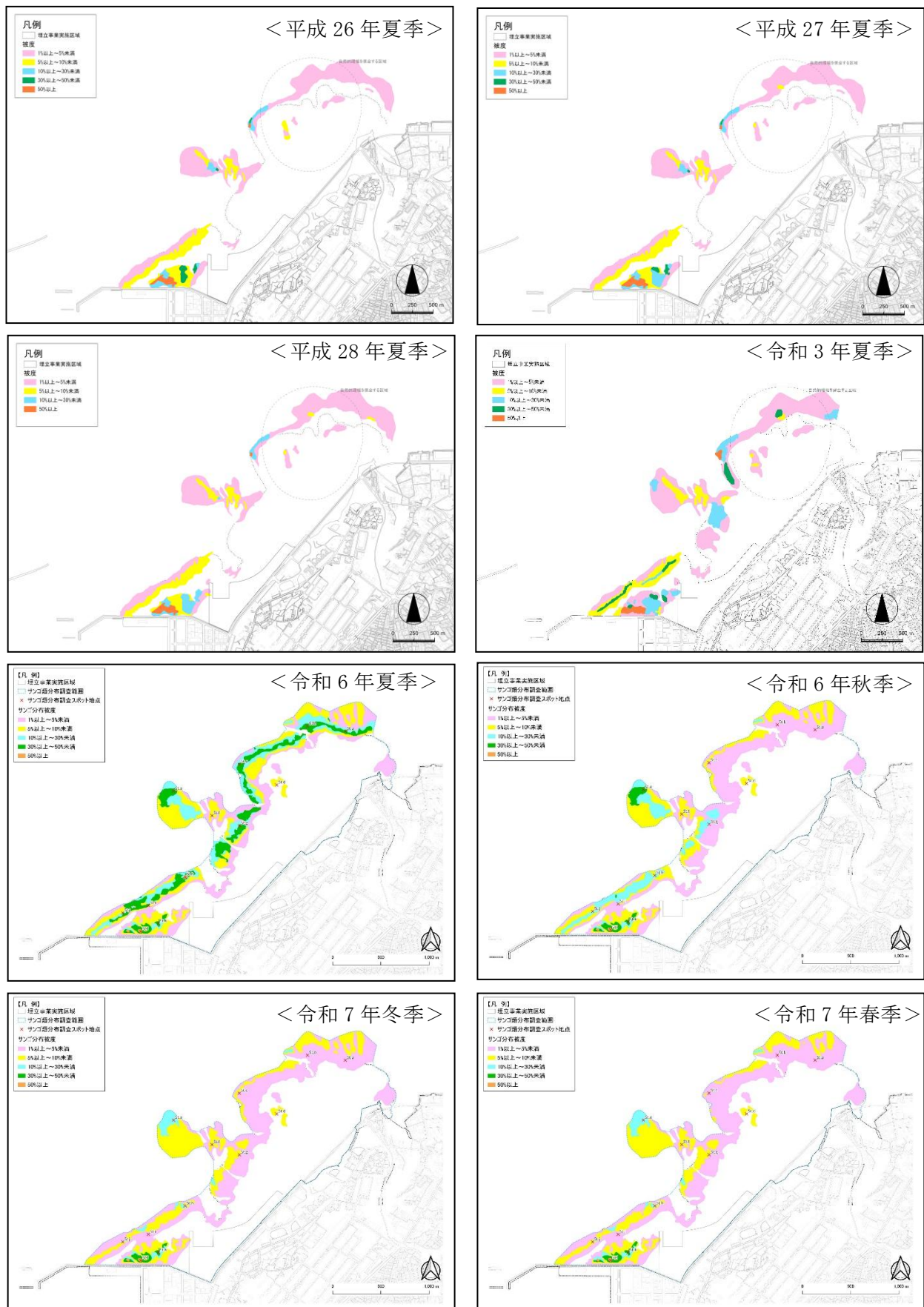
図 6.12.23 サンゴ分布域の変遷
