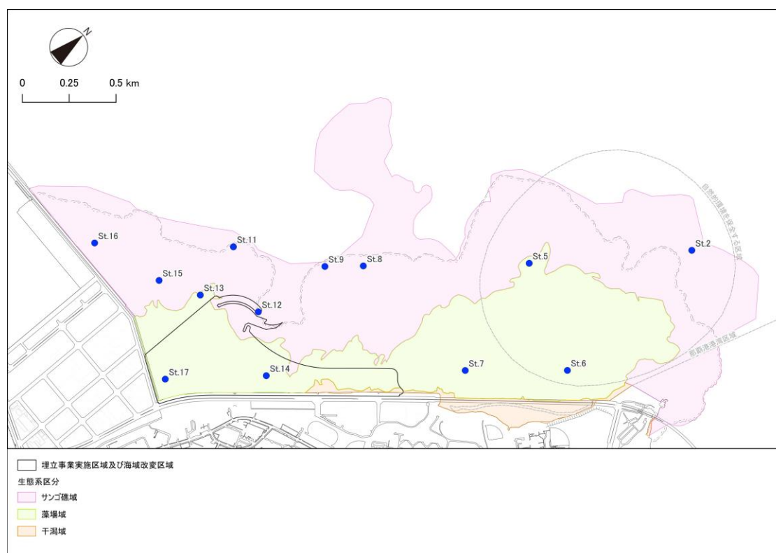
図 6.12.34 底生動物の推定に用いた調査地点 (St. 12、14、17)
