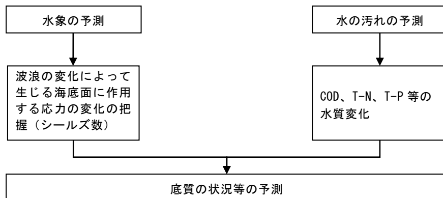
図 6.8.2.4 埋立地の存在時の底質の状況等の予測手順
