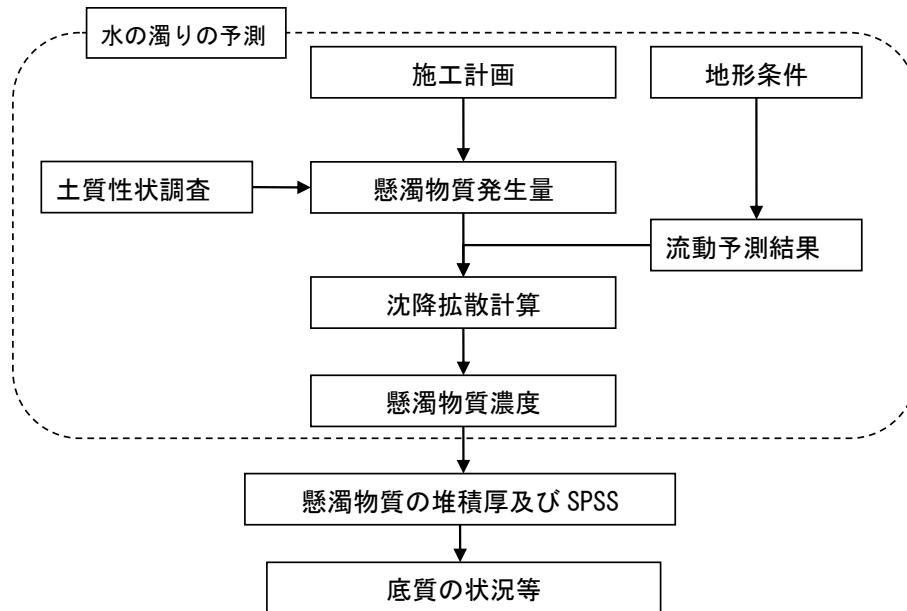
図 6.8.2.1 工事の実施に伴う底質の状況等の予測手順
