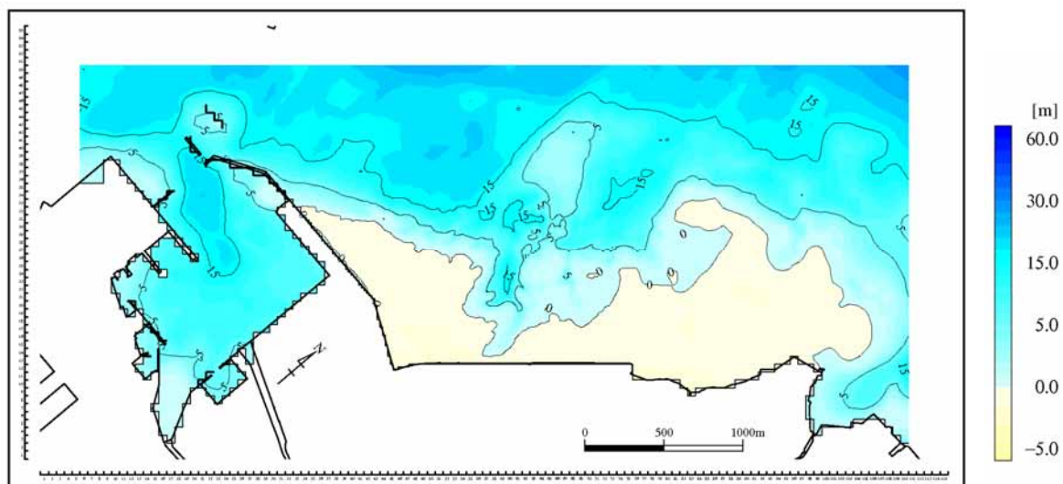
図 6.5.2.25(3) 計算範囲とその水深（単位：m DL 基準、中領域：50m 格子）
