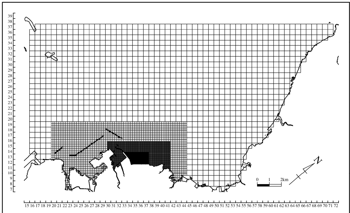
図 6.5.2.26(1) 計算範囲の格子分割（緩衝領域：450m 格子）
