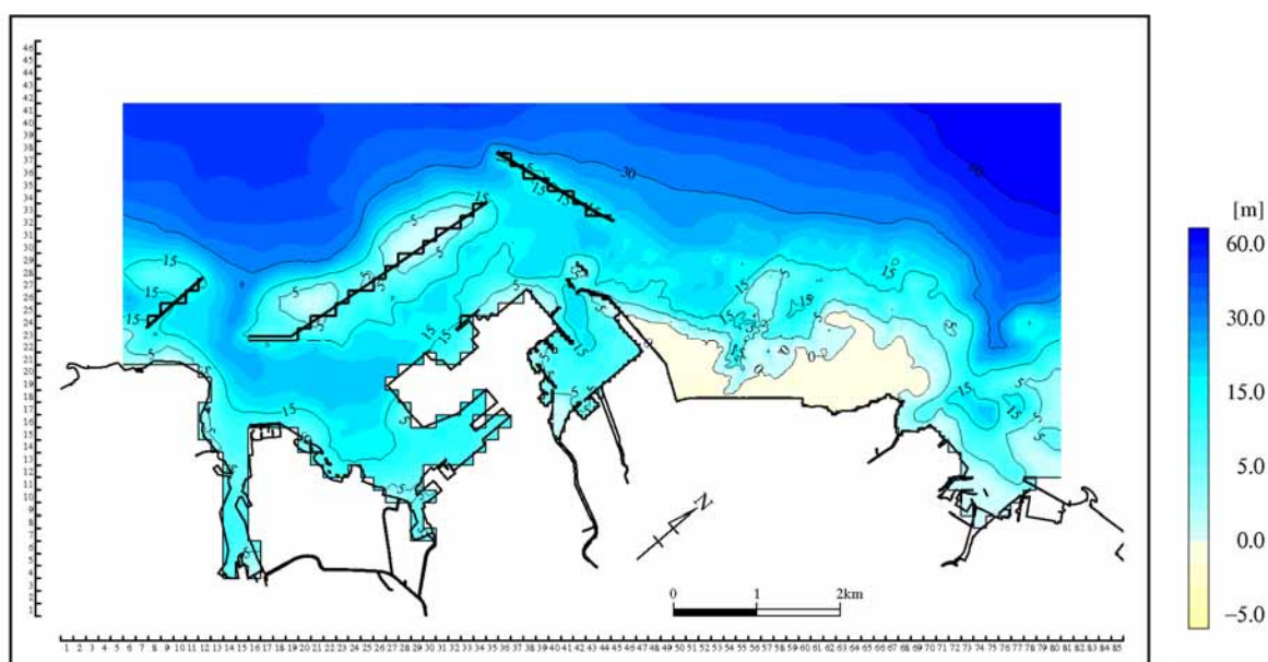
図 6.5.2.25(2) 計算範囲とその水深（単位：m DL 基準、大領域：150m 格子）
