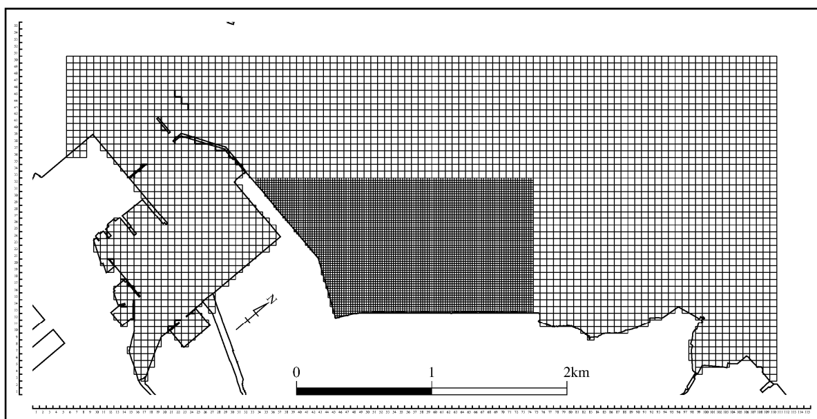
図 6.5.2.26(3) 計算範囲の格子分割（中領域：50m 格子）
