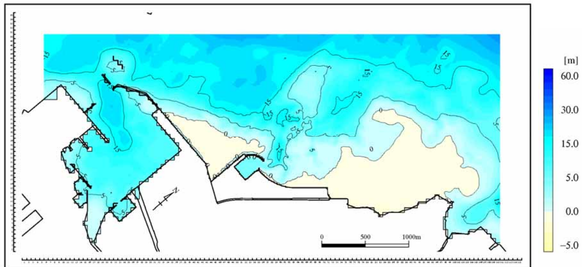
図 6.5.2.31(1) 存在時予測に用いた地形図及び水深図 (単位 : m DL 基準、中領域 : 50m 格子)
