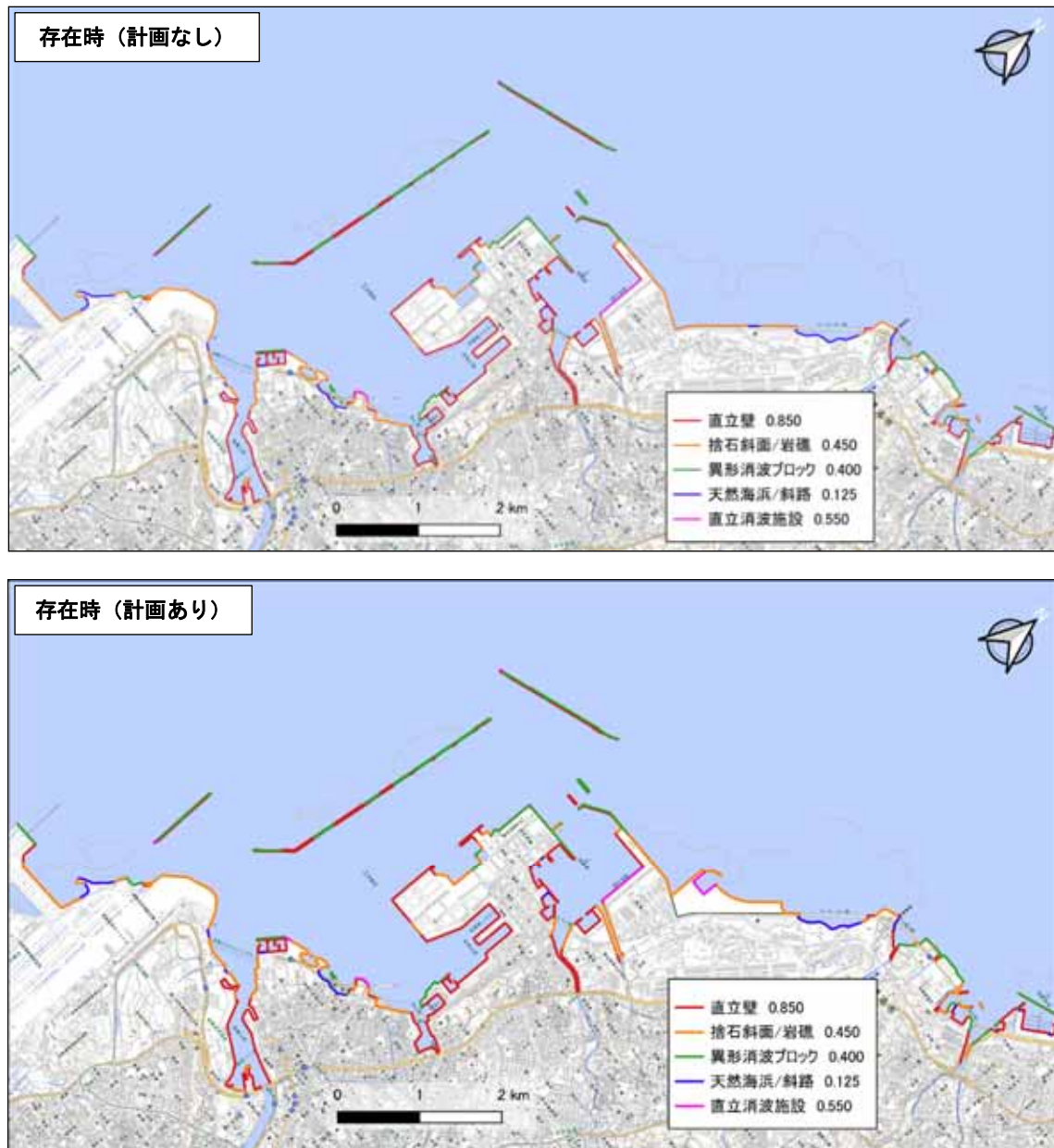
図 6.5.2.21 存在時（計画なし、計画あり）の反射率設定図
