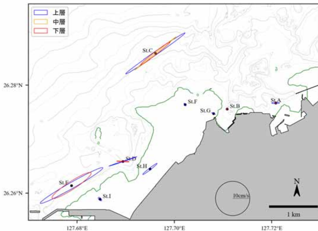
図 6.5.1.11(1) 主要 4 分潮の潮流楕円の平面分布図 ( M_2 分潮、夏季)
