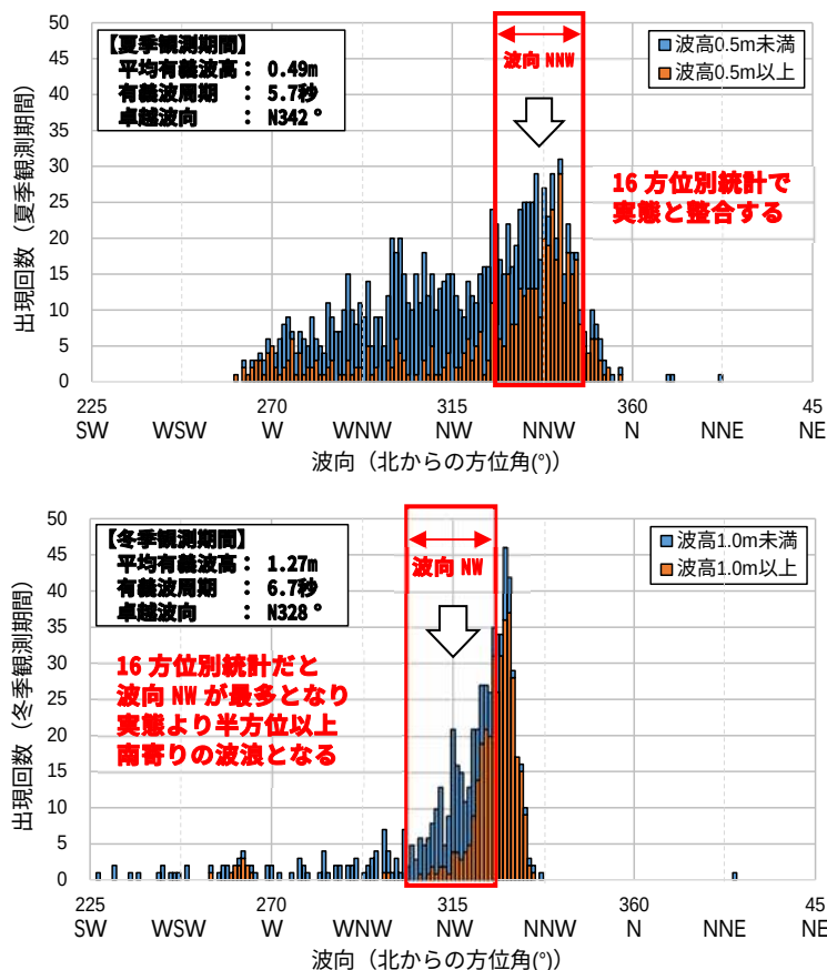
図 6.5.1.8 St.C の波向出現頻度 [角度] (夏季、冬季)
