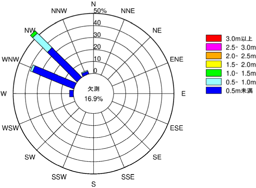
図 6.5.1.2(2) 波高と波向の出現頻度分布（夏季、St.D）
