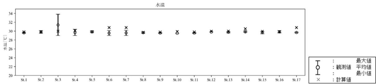
図 6.5.2.38(1) 観測値と計算値との比較（水温[°C]、夏季）
