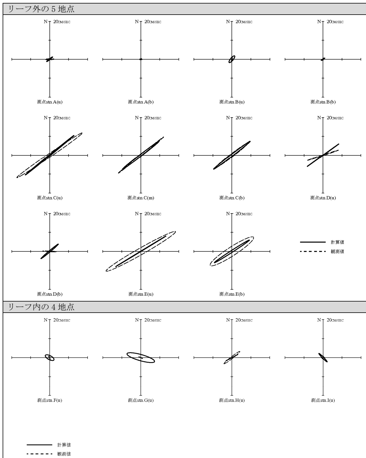
図 6.5.2.34 潮流楕円の比較（夏季）
