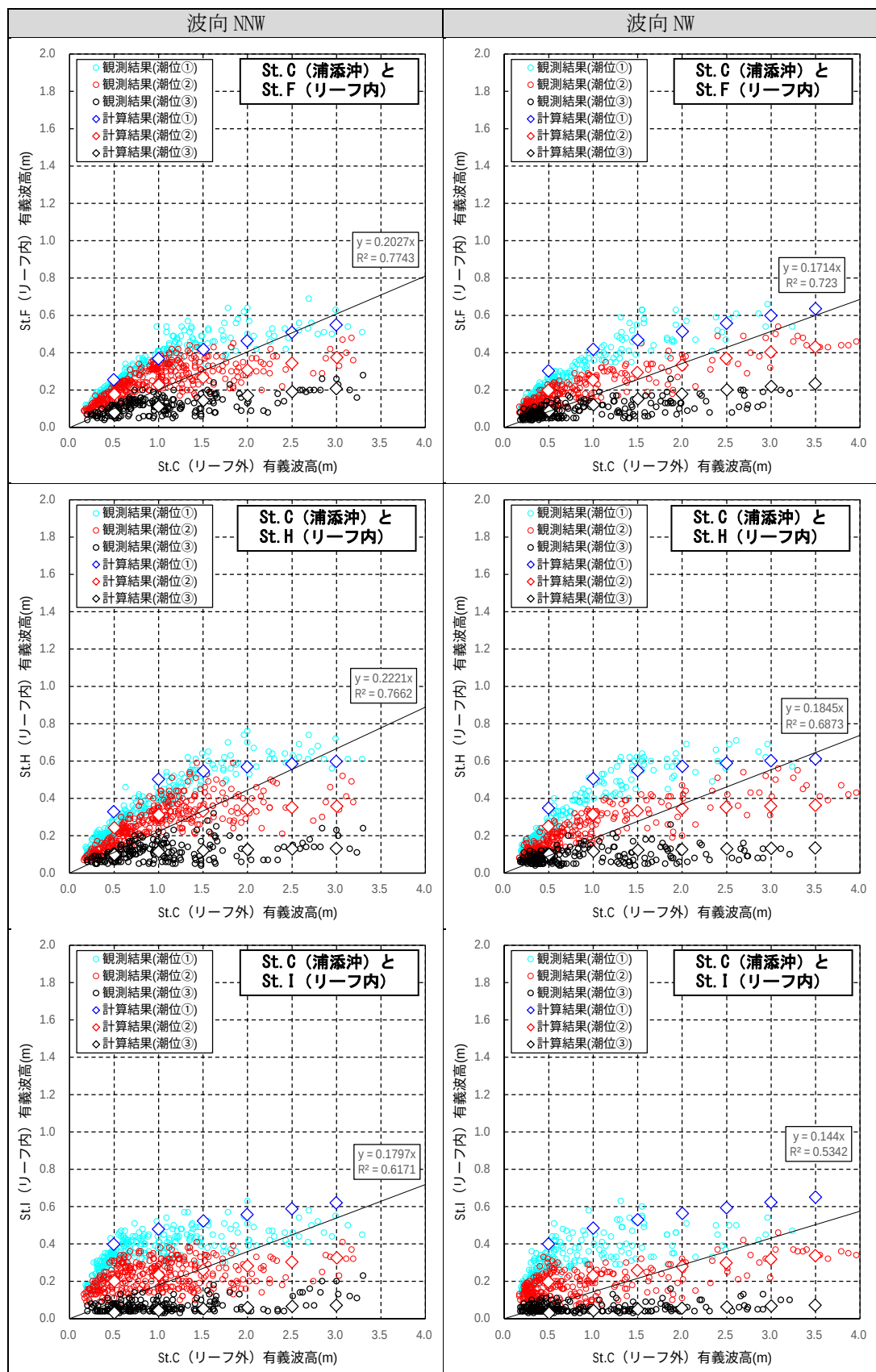
図 6.5.2.16 浦添沖 (St.C) とリーフ内の波浪観測地点における波高の散布図
