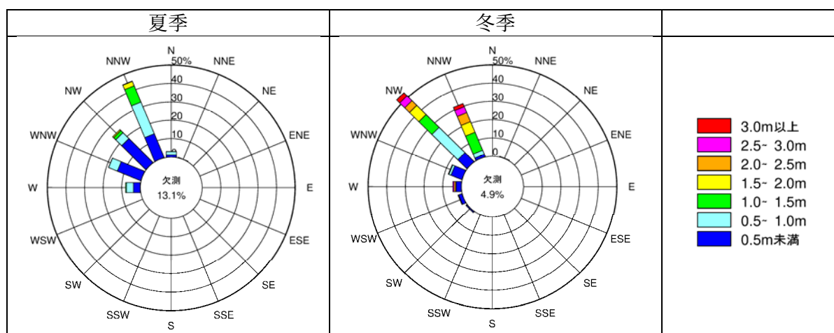
図 6.5.1.7 St.C の波向出現頻度 [方位] (夏季、冬季)
