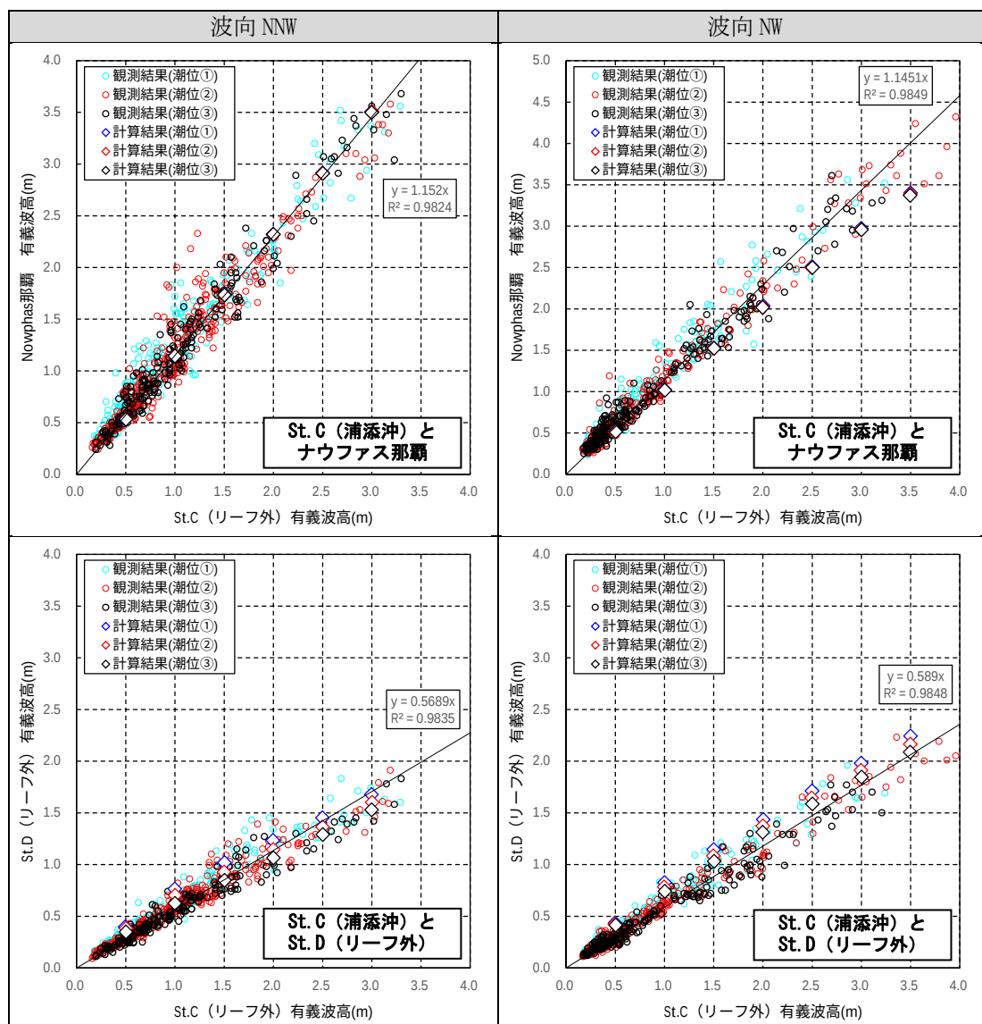
図 6.5.2.15 浦添沖(St. C)とリーフ外の波浪観測地点における波高の散布図
