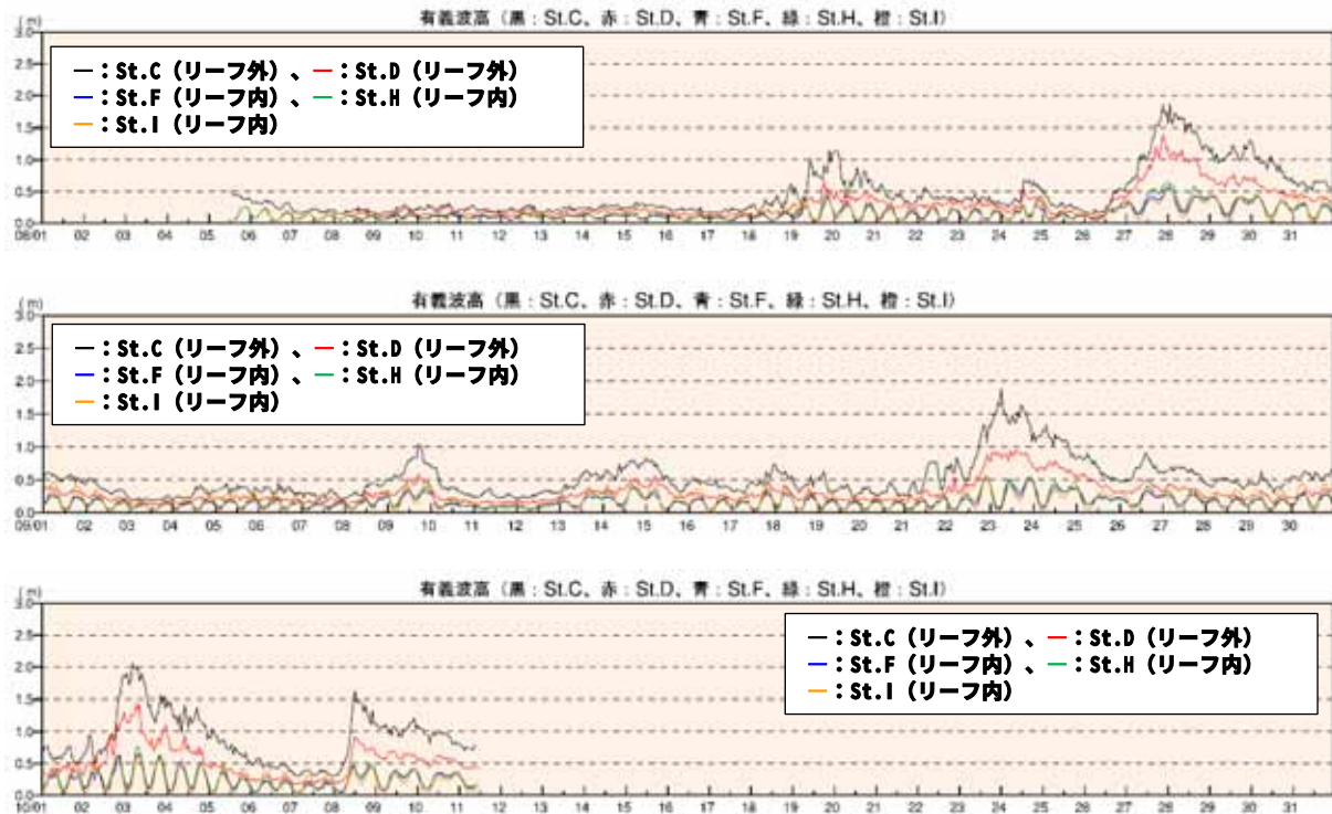
図 6.5.1.4(1) 各地点の有義波高の時系列の比較 (夏季 (令和 6 年 8 月～10 月))
