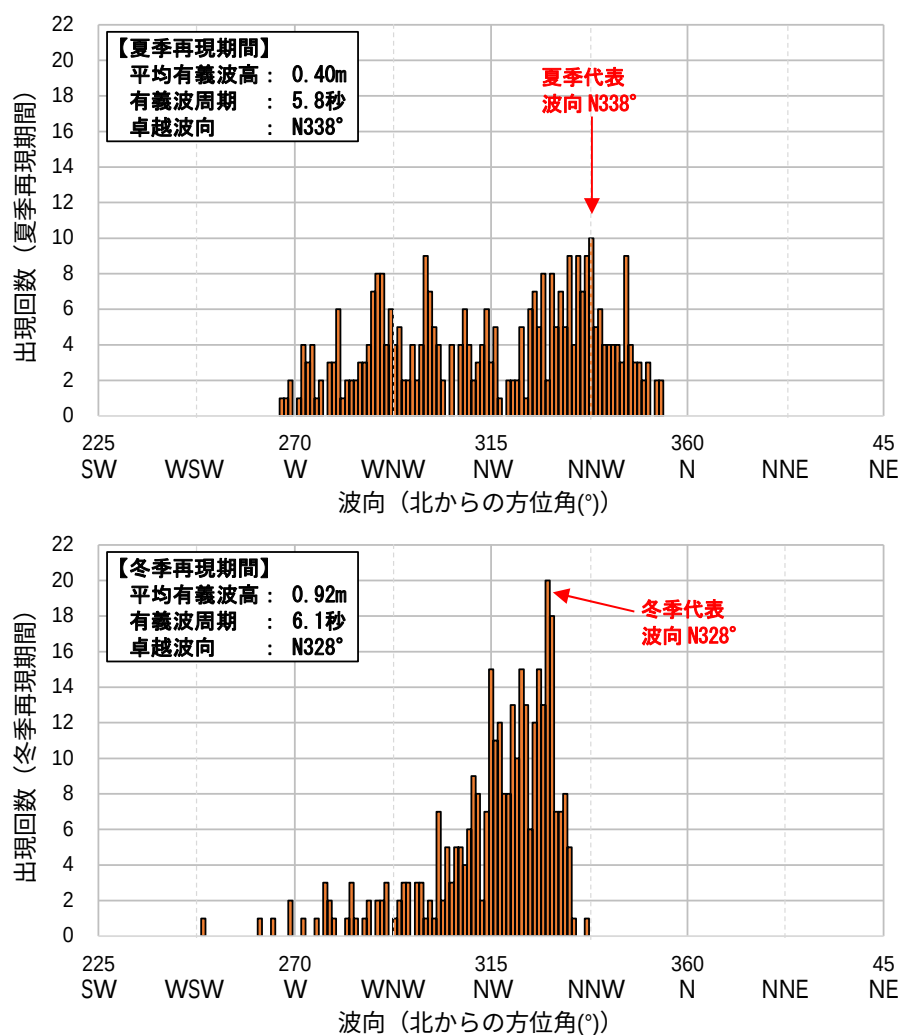
図 6.5.2.17 浦添沖(St. C)における再現期間の波向出現状況（再現期間は表 6.5.2.7 参照）
