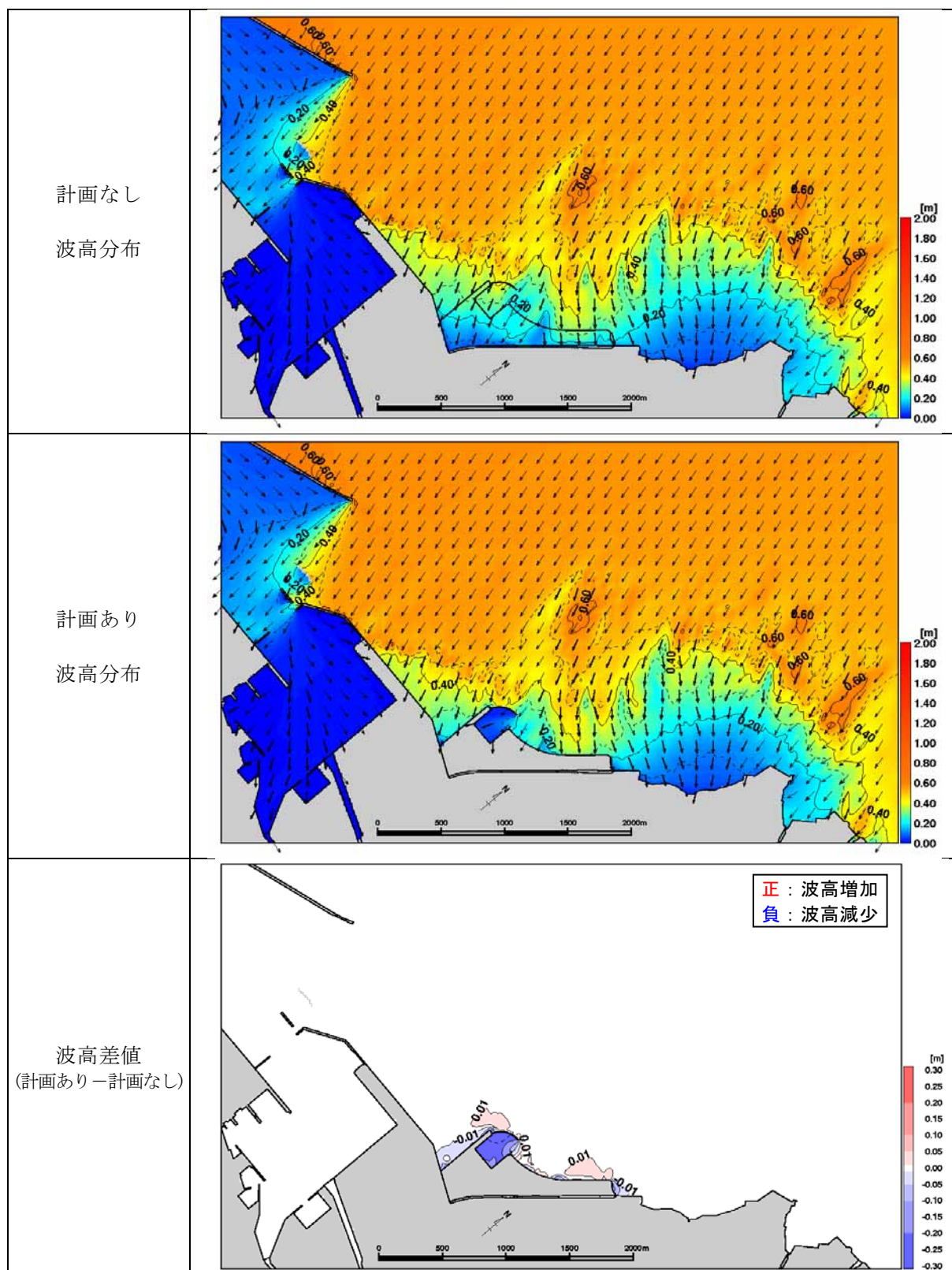
図 6.5.2.46(1) 波高分布（夏季、平常時、平均大潮潮、平均高潮位 (M. H. W. L. )）
