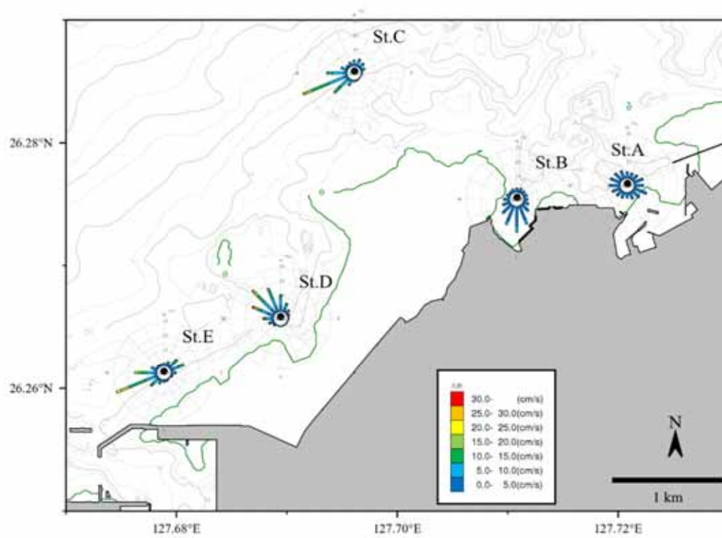
图 6.5.1.10(3) 流向・流速頻度分布(冬季、下層)
