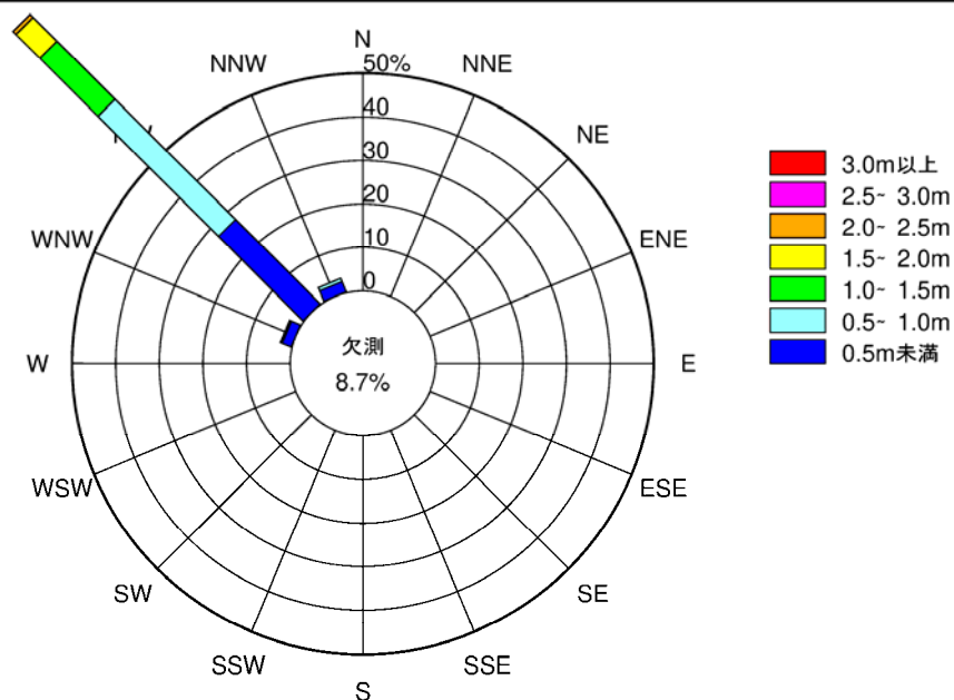
図 6.5.1.3(2) 波高と波向の出現頻度分布 (冬季、St.D)
