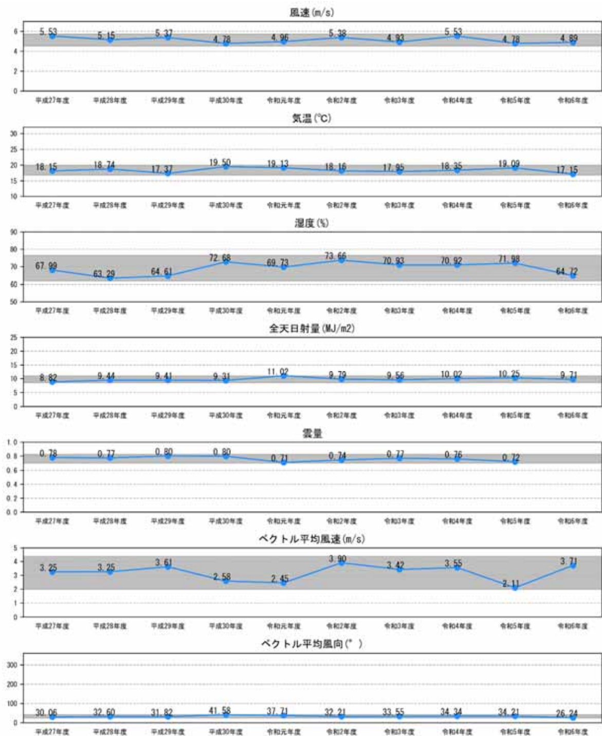
図 6.5.2.30(2) 潮流調査期間を含む近年10か年度の気象条件平均値の比較（冬季）
