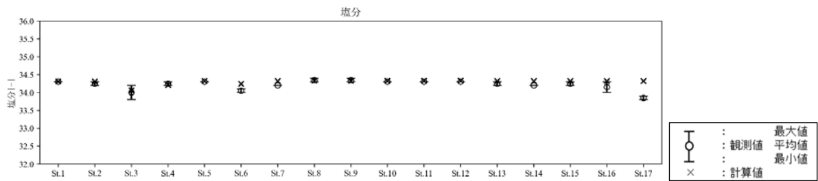
図 6.5.2.38(2) 観測値と計算値との比較（塩分[-]、夏季）
