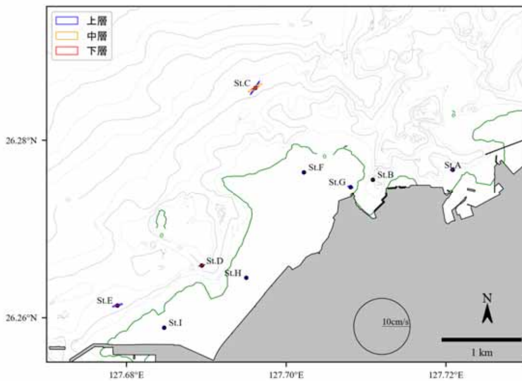
図 6.5.1.11(3) 主要 4 分潮の潮流橢円の平面分布図 ( K_1 分潮、夏季)
