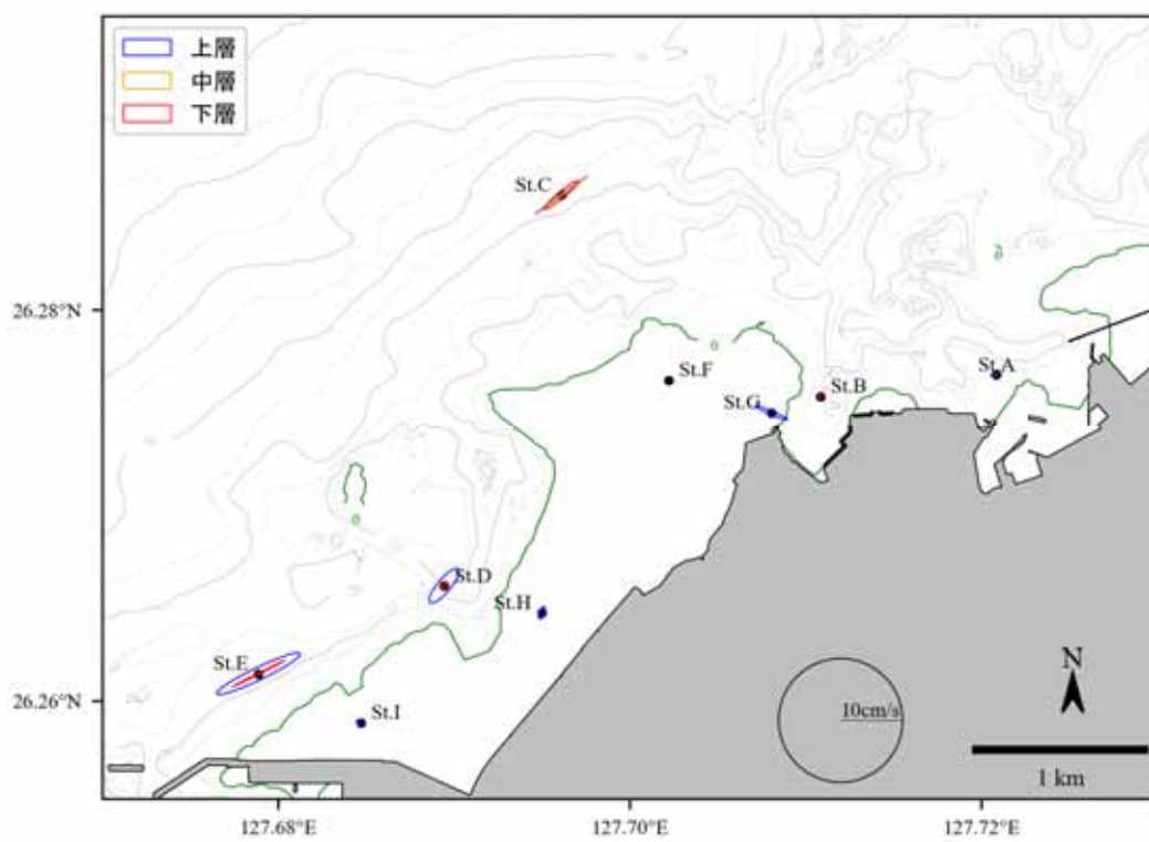
図 6.5.1.12(2) 主要 4 分潮の潮流楕円の平面分布図 ( S_2 分潮、冬季)
