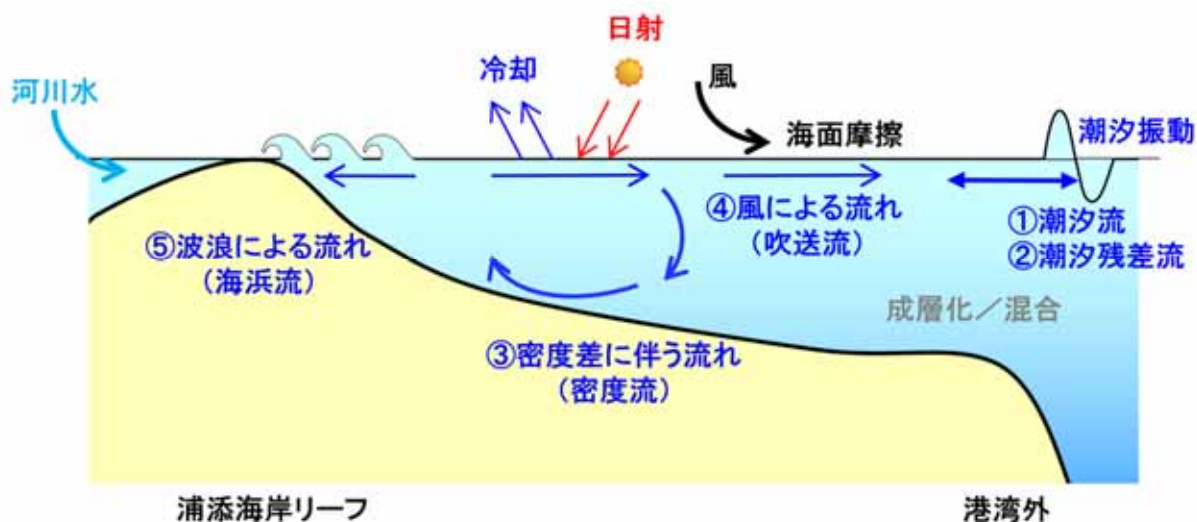
図 6.5.2.24 流動モデルが解析する主な現象
