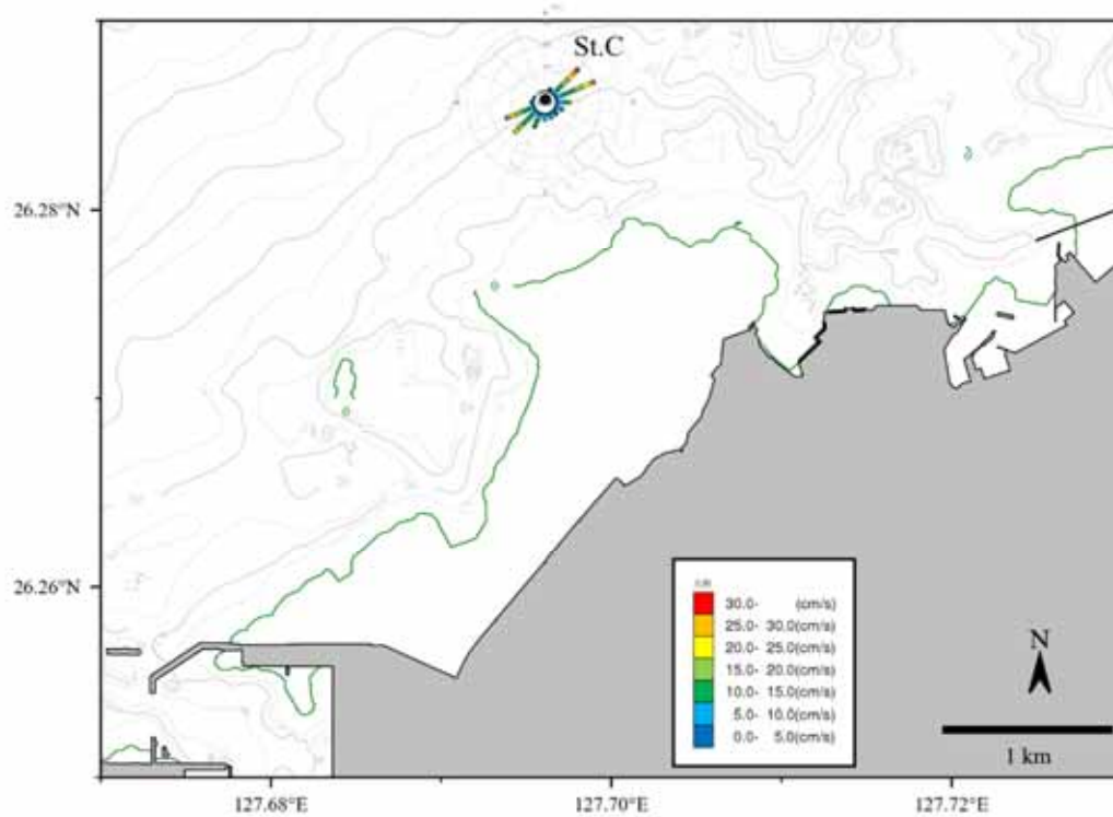
图 6.5.1.9(2) 流向・流速頻度分布(夏季、中層)
