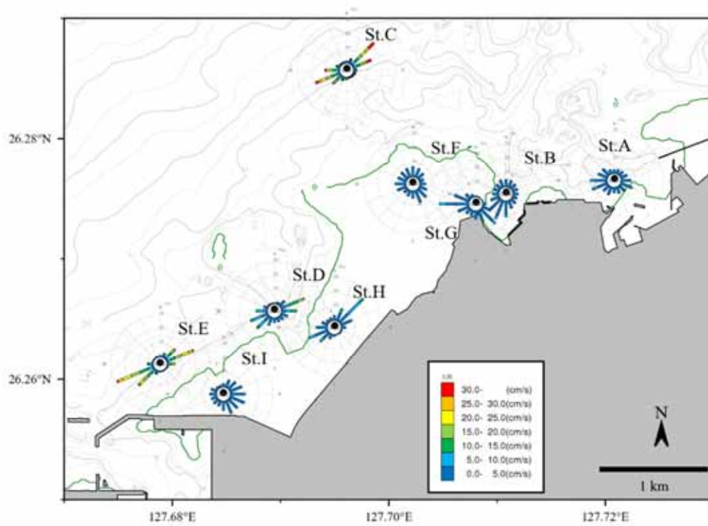
图 6.5.1.9(1) 流向・流速頻度分布(夏季、上層)
