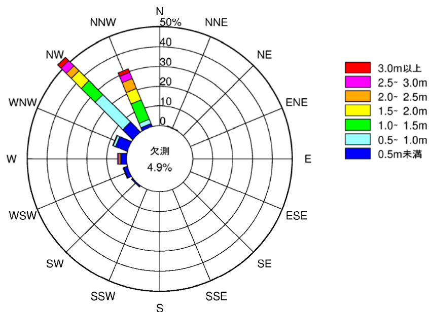
図 6.5.1.3(1) 波高と波向の出現頻度分布 (冬季、St.C)
