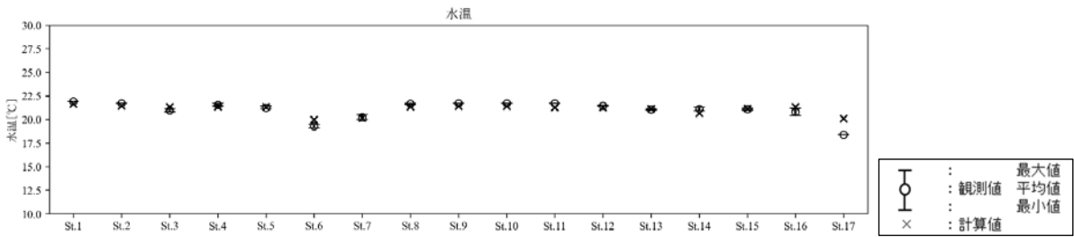
図 6.5.2.39(1) 観測値と計算値との比較（水温[°C]、冬季）
