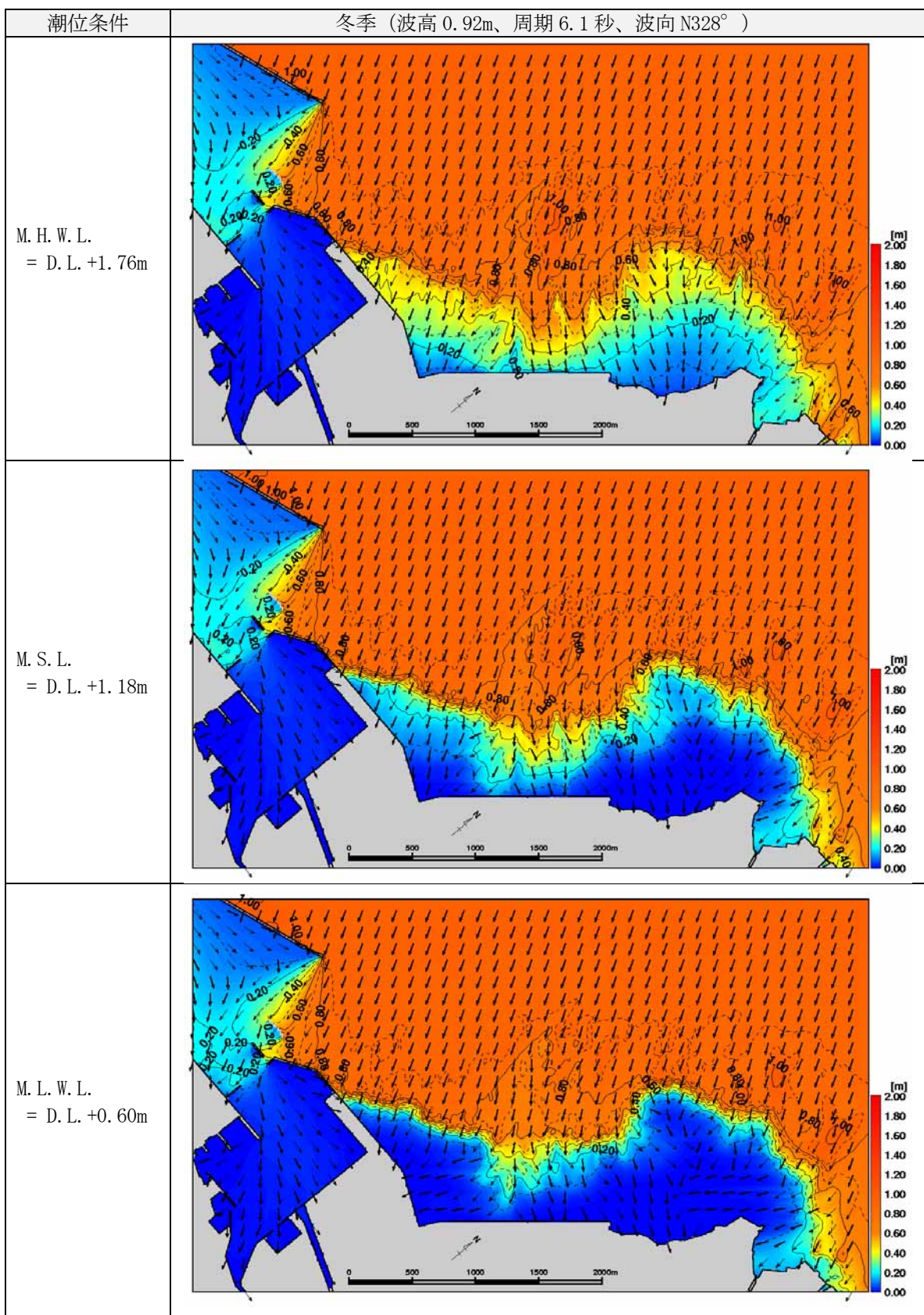
図 6.5.2.19 波高分布 (冬季) (浦添沖の波浪条件 波高：0.92m、周期：6.1s、波向：N328° )
