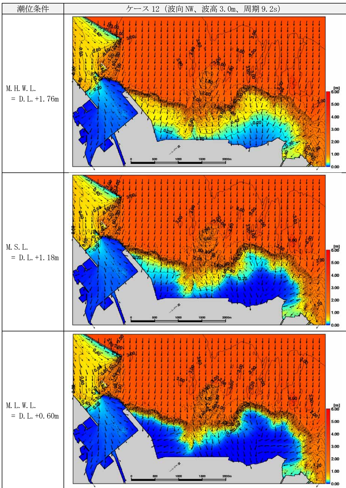
図 6.5.2.13 波高・波向分布図 (表 6.5.2.5 のケース 12)
