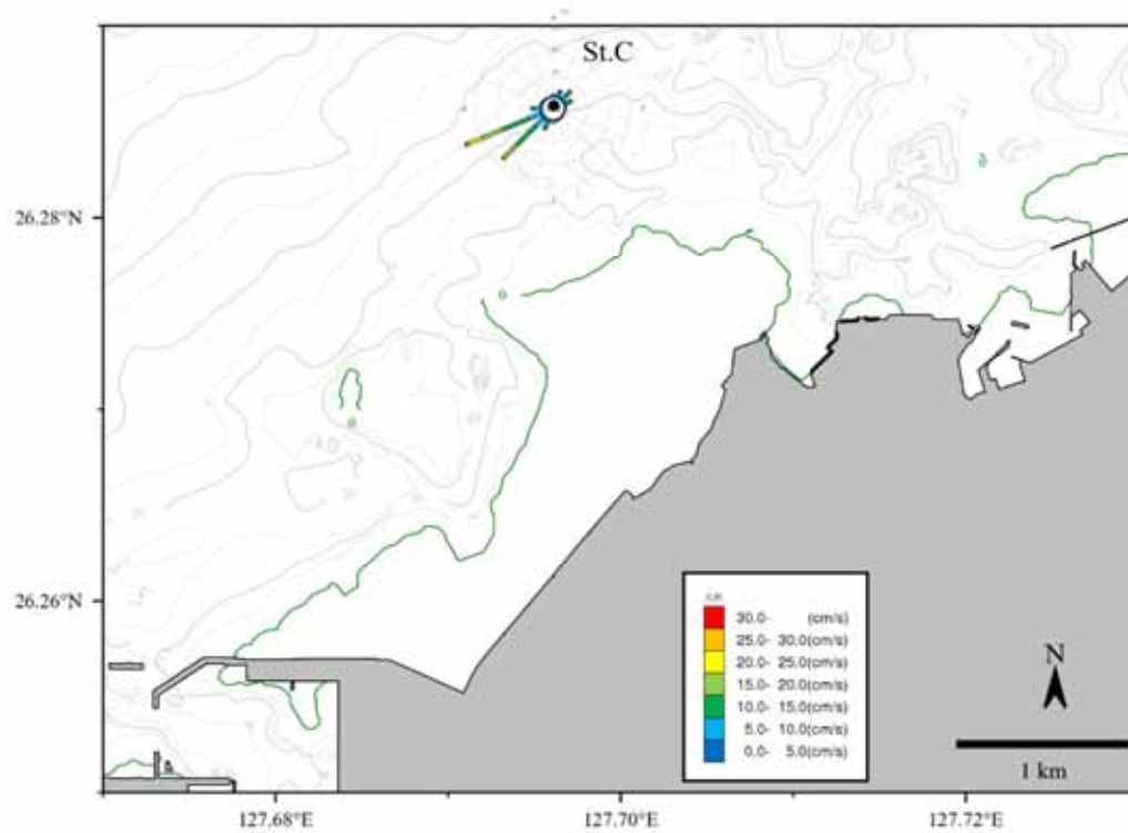
图 6.5.1.10(2) 流向・流速頻度分布(冬季、中層)
