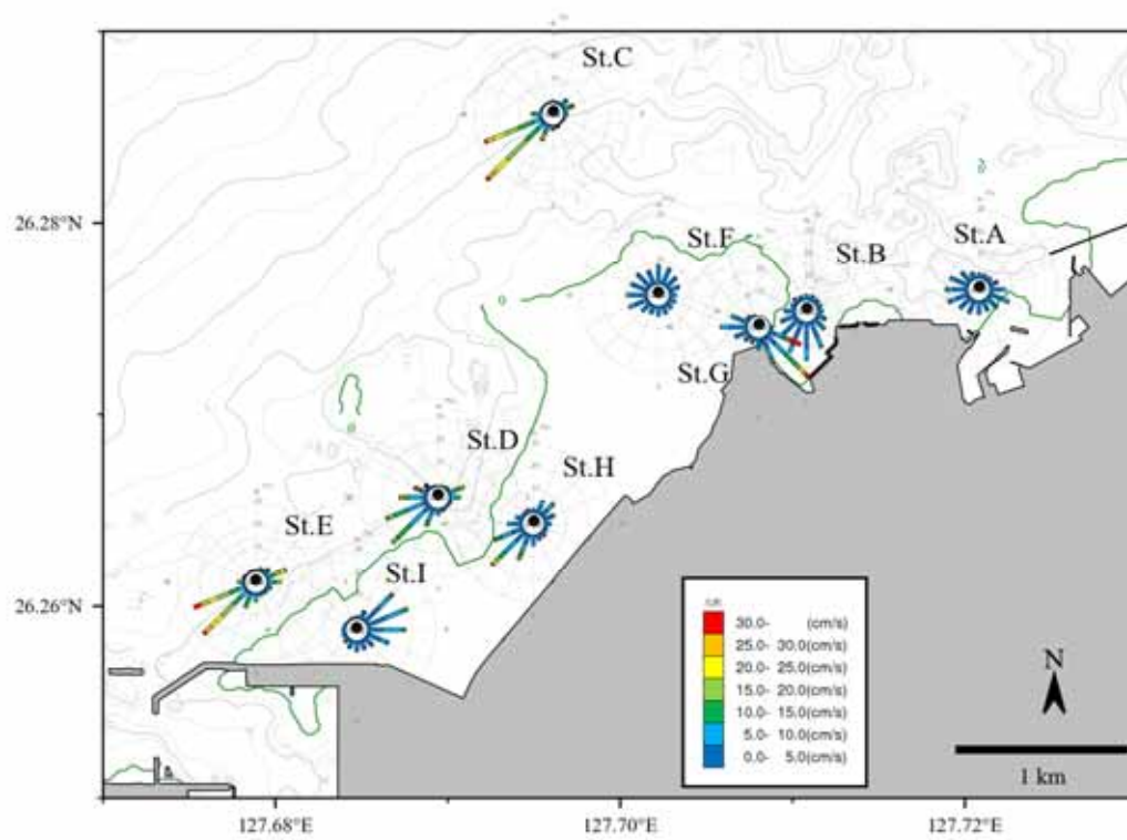
图 6.5.1.10(1) 流向・流速頻度分布(冬季、上層)
