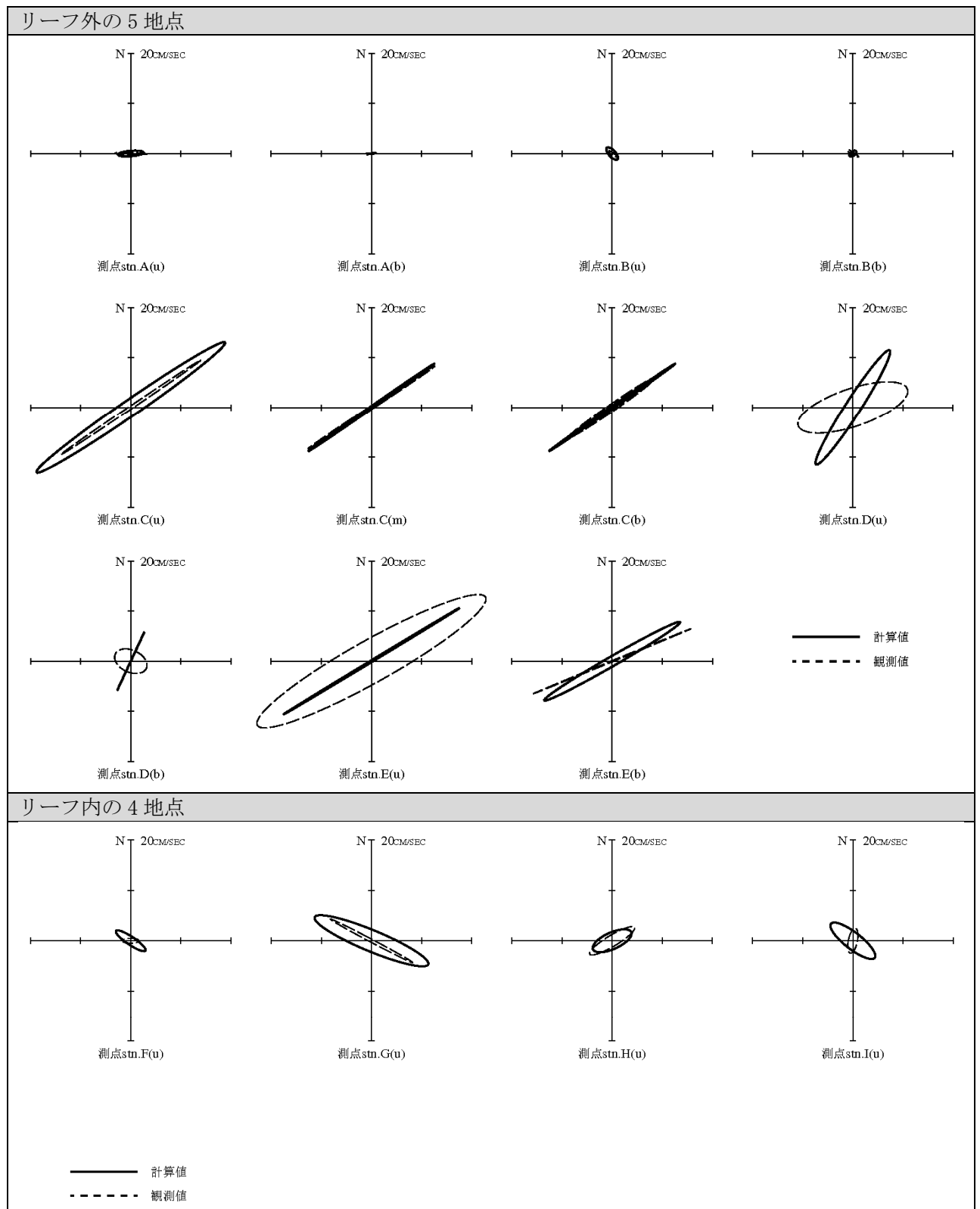
図 6.5.2.41 冬季における平均大潮期流況のホドグラフの比較
