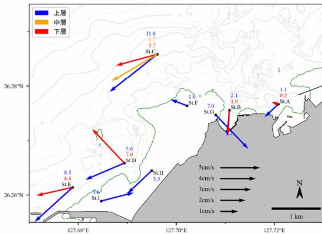
图 6.5.1.16 平均流分布 (冬季)
