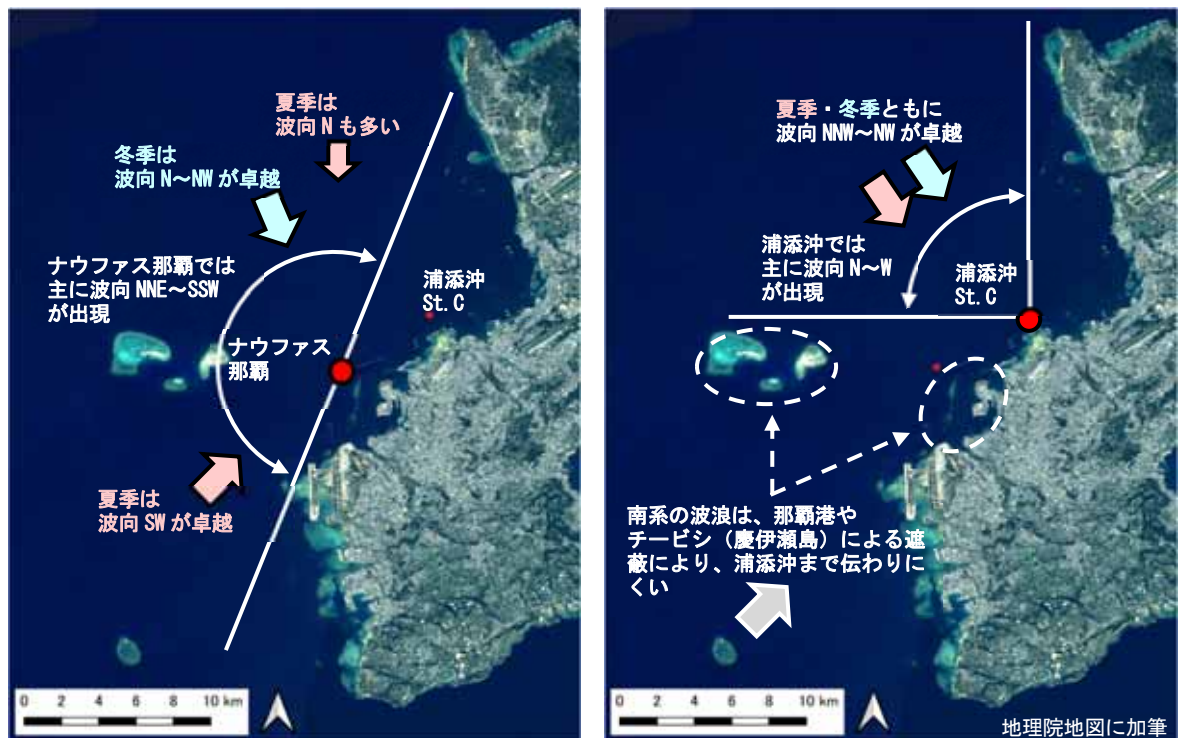
図 6.5.2.7 ナウファス那覇及び浦添沖 St. C における波浪特性
