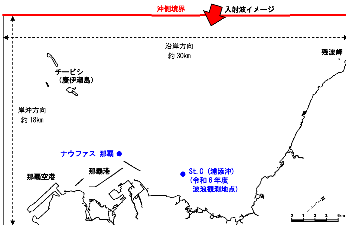
図 6.5.2.4 波浪計算の計算領域と主な波浪観測地点
