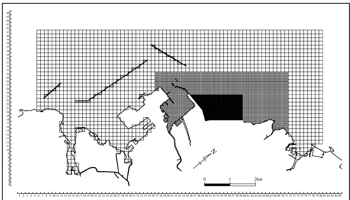
図 6.5.2.26(2) 計算範囲の格子分割（大領域：150m 格子）
