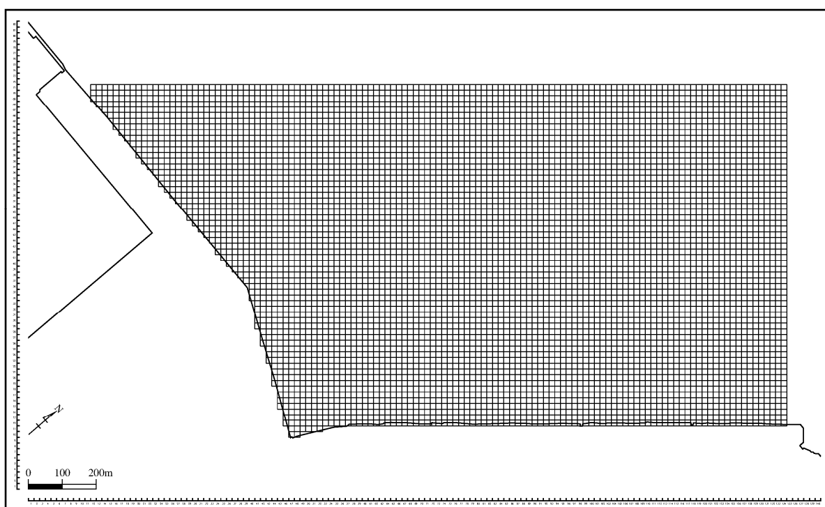
図 6.5.2.26(4) 計算範囲の格子分割（小領域：16.7m 格子）
