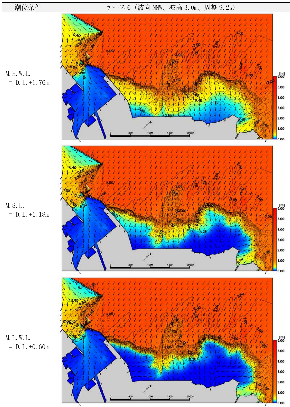
図 6.5.2.12 波高・波向分布図 (表 6.5.2.5 のケース 6)
