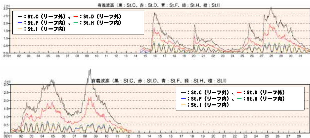
図 6.5.1.4(2) 各地点の有義波高の時系列の比較 (冬季 (令和 7 年 1 月～2 月))
