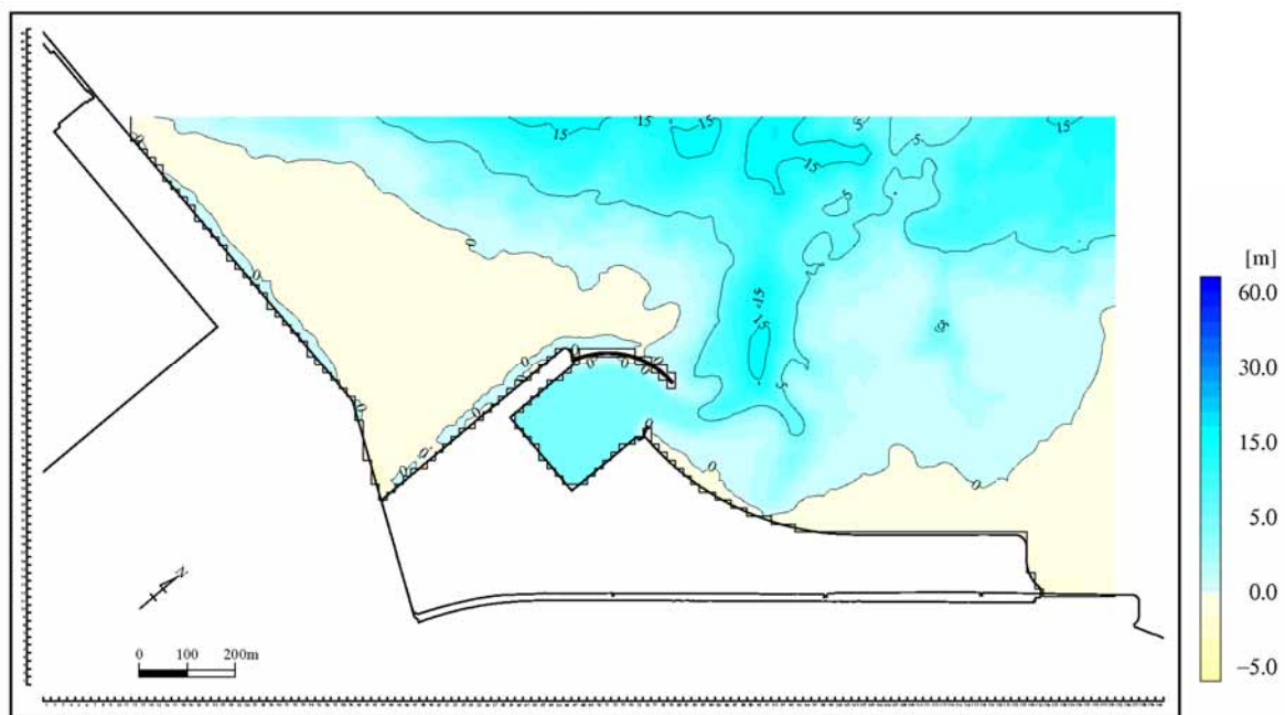
図 6.5.2.31(2) 存在時予測に用いた地形図及び水深図 (単位 : m DL 基準、小領域 : 16.7m 格子)
