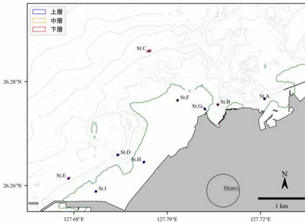
図 6.5.1.12(4) 主要 4 分潮の潮流橢円の平面分布図 ( O_1 分潮、冬季)
