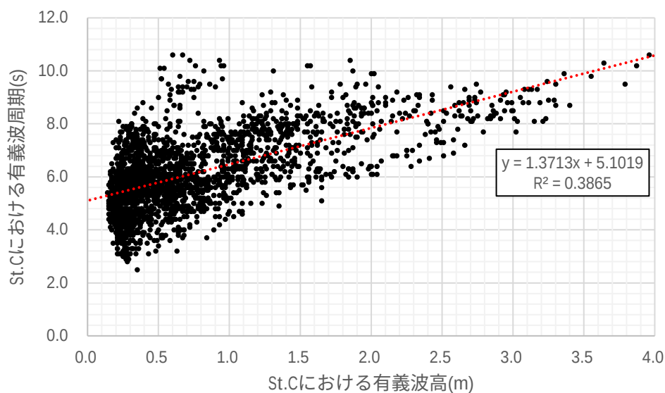
図 6.5.2.11 浦添沖(St.C)における有義波高と有義波周期の関係
