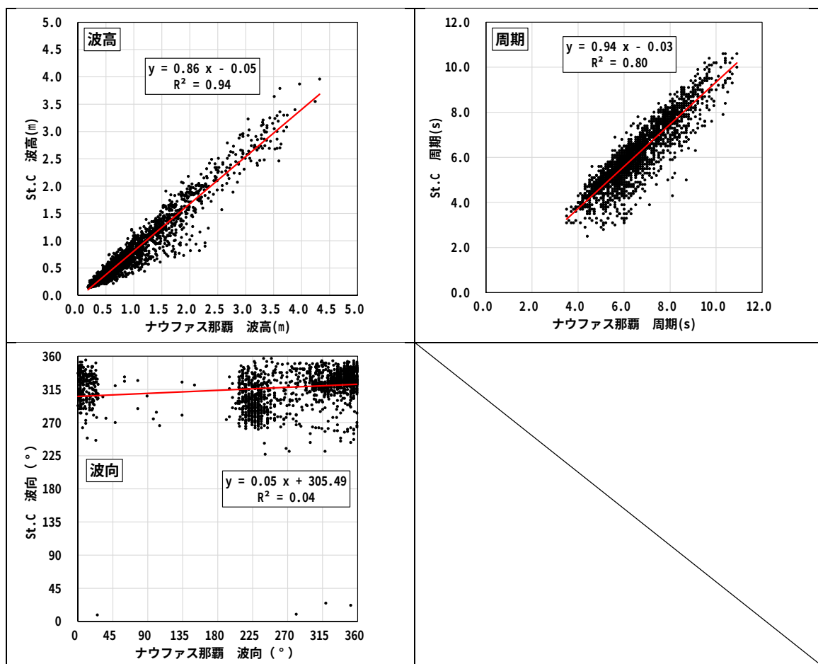
図 6.5.1.6 ナウファス那覇と St.C の波浪（波高、周期、波向）の関係
