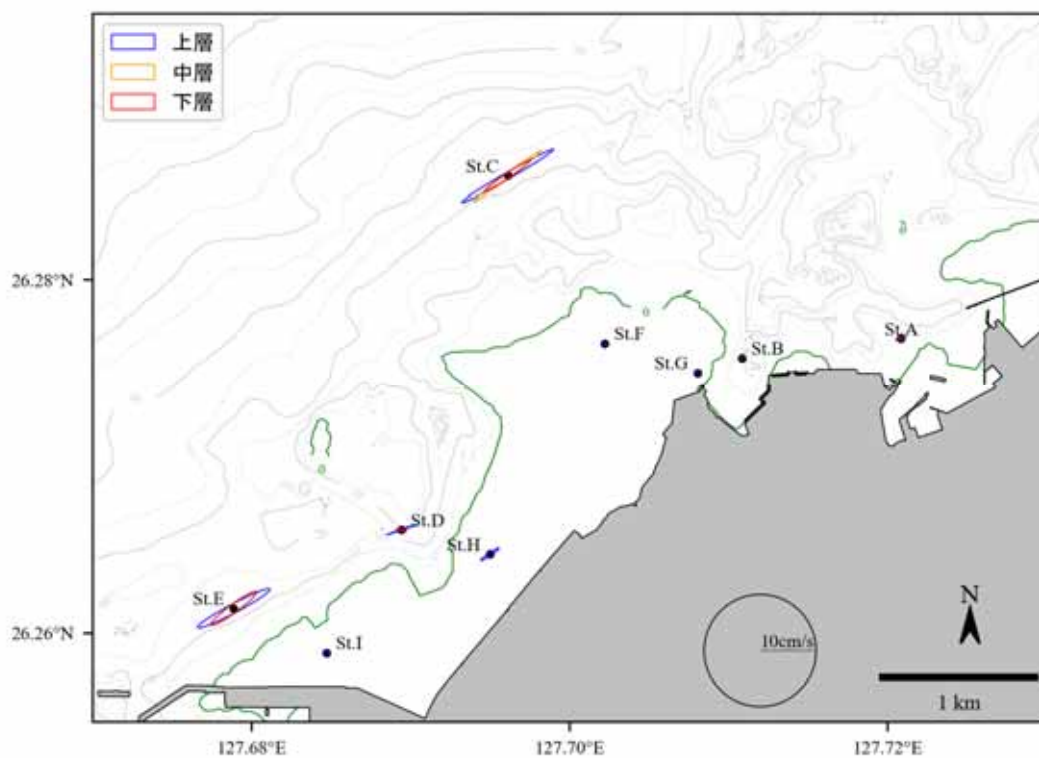
図 6.5.1.11(2) 主要 4 分潮の潮流楕円の平面分布図 ( S_2 分潮、夏季)
