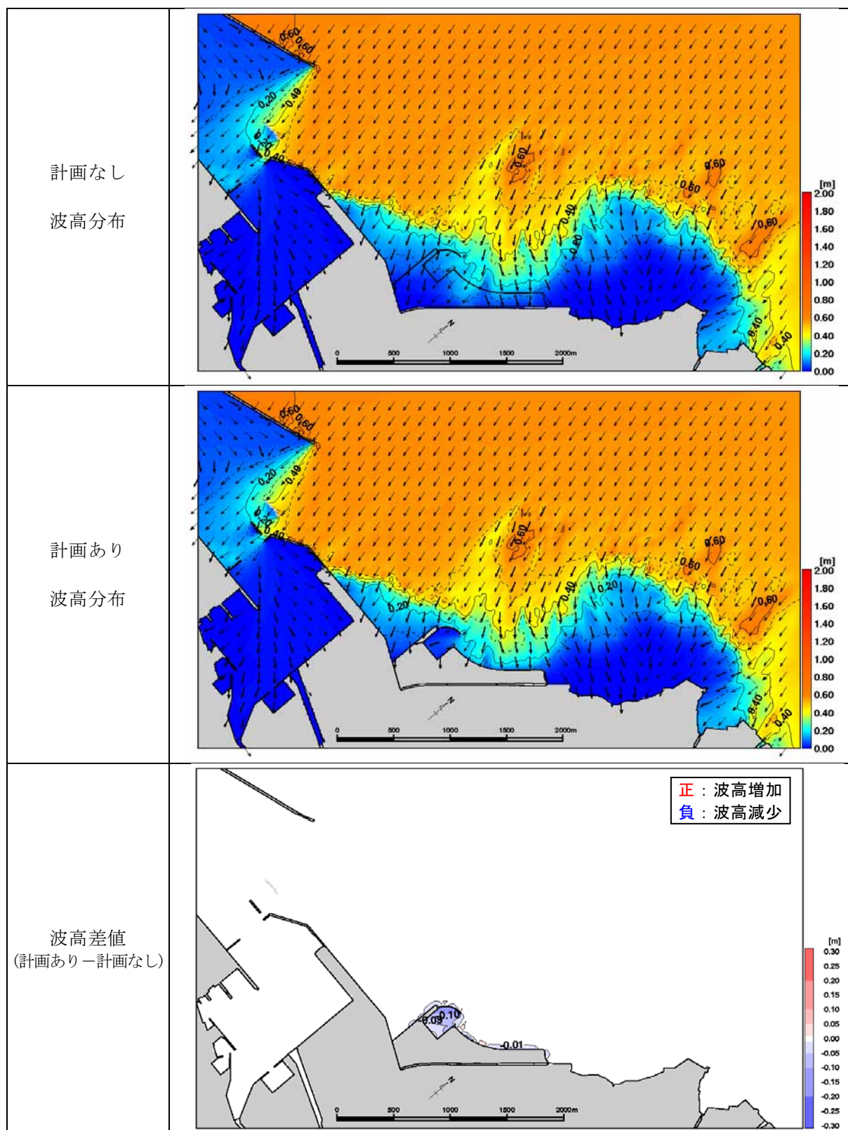
図 6.5.2.46(2) 波高分布（夏季、平常時、平均大潮潮、平均潮位(M. S. L.))
