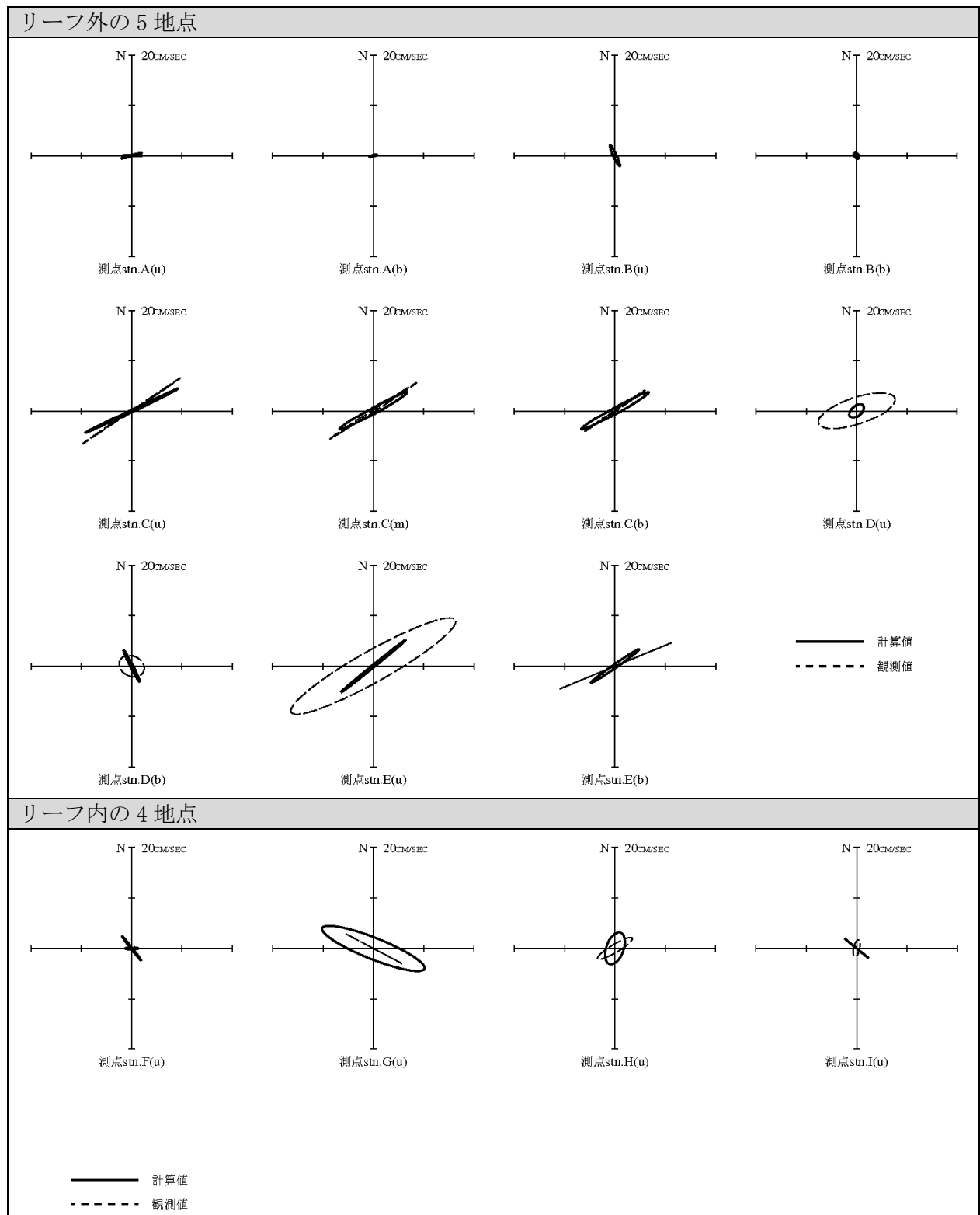
図 6.5.2.35 潮流楕円の比較（冬季）
