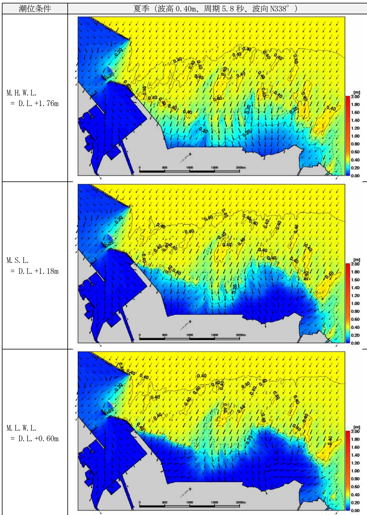
図 6.5.2.18 波高分布 (夏季) (浦添沖の波浪条件 波高：0.40m、周期：5.8s、波向：N338° )
