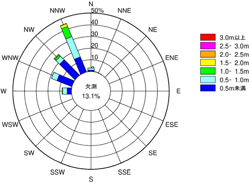
図 6.5.1.2(1) 波高と波向の出現頻度分布（夏季、St.C）
