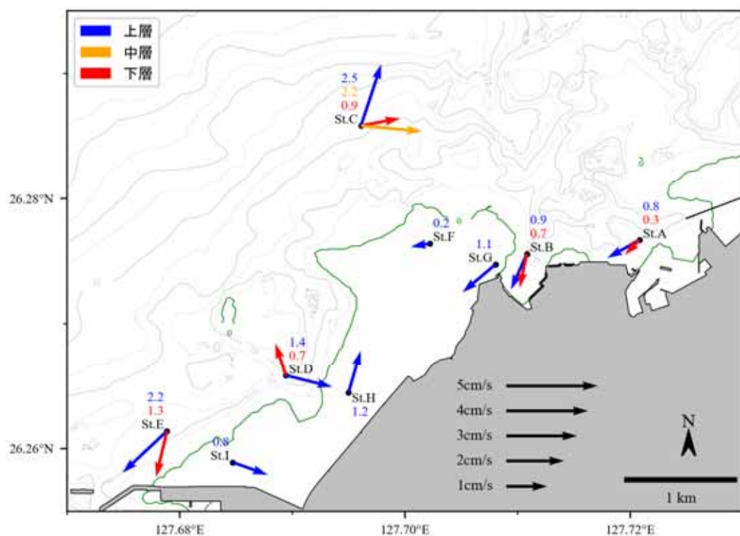
图 6.5.1.15 平均流分布 (夏季)
