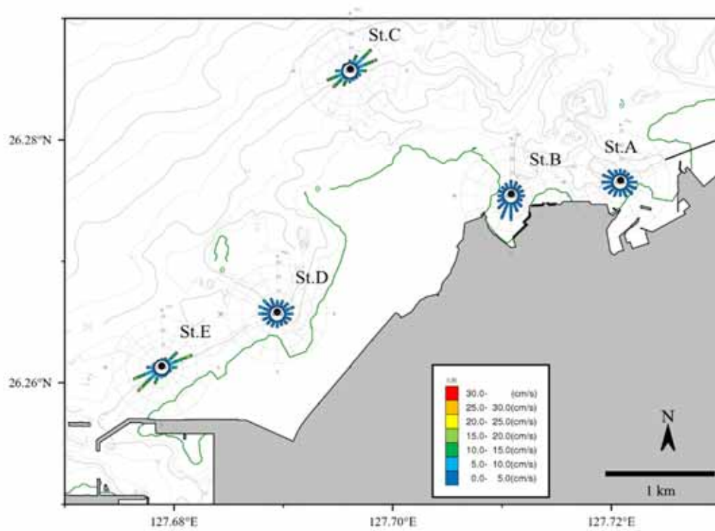
図 6.5.1.9(3) 流向・流速頻度分布(夏季、下層)
