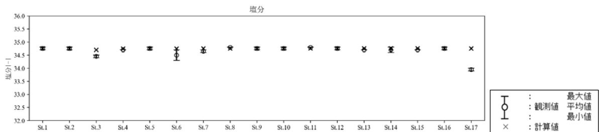
図 6.5.2.39(2) 観測値と計算値との比較（塩分[-]、冬季）
