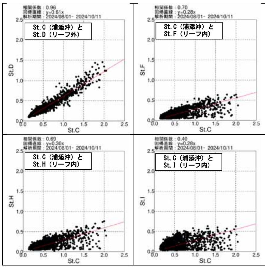
図 6.5.2.9 浦添沖の St.C とリーフ内外の St.D, F, H, I の各地点の波高の比較（全観測期間）
