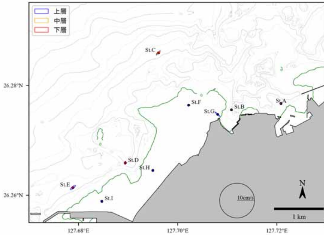
図 6.5.1.12(3) 主要 4 分潮の潮流橢円の平面分布図 ( K_1 分潮、冬季)
