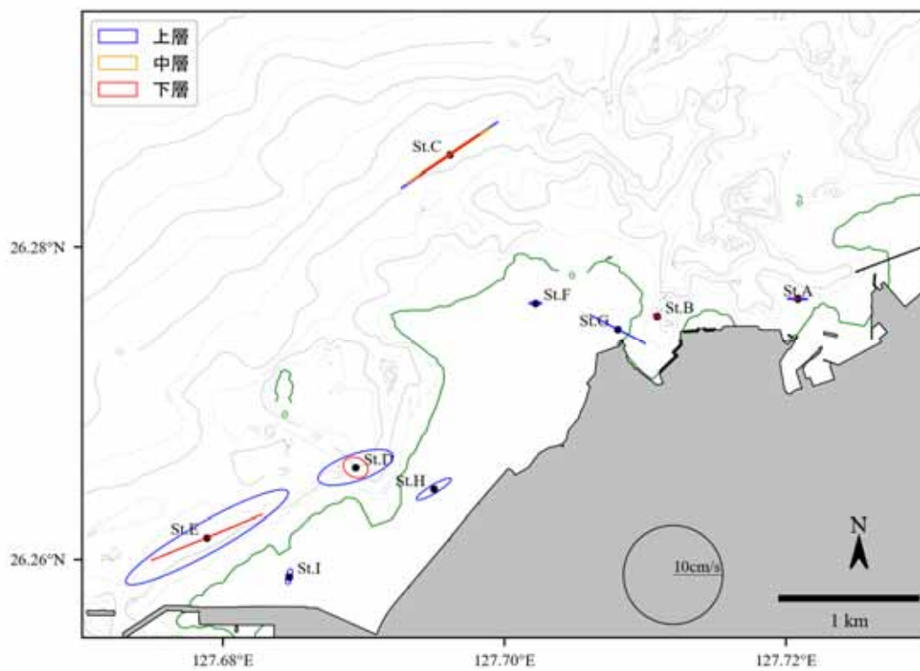
図 6.5.1.12(1) 主要 4 分潮の潮流楕円の平面分布図 ( M_2 分潮、冬季)
