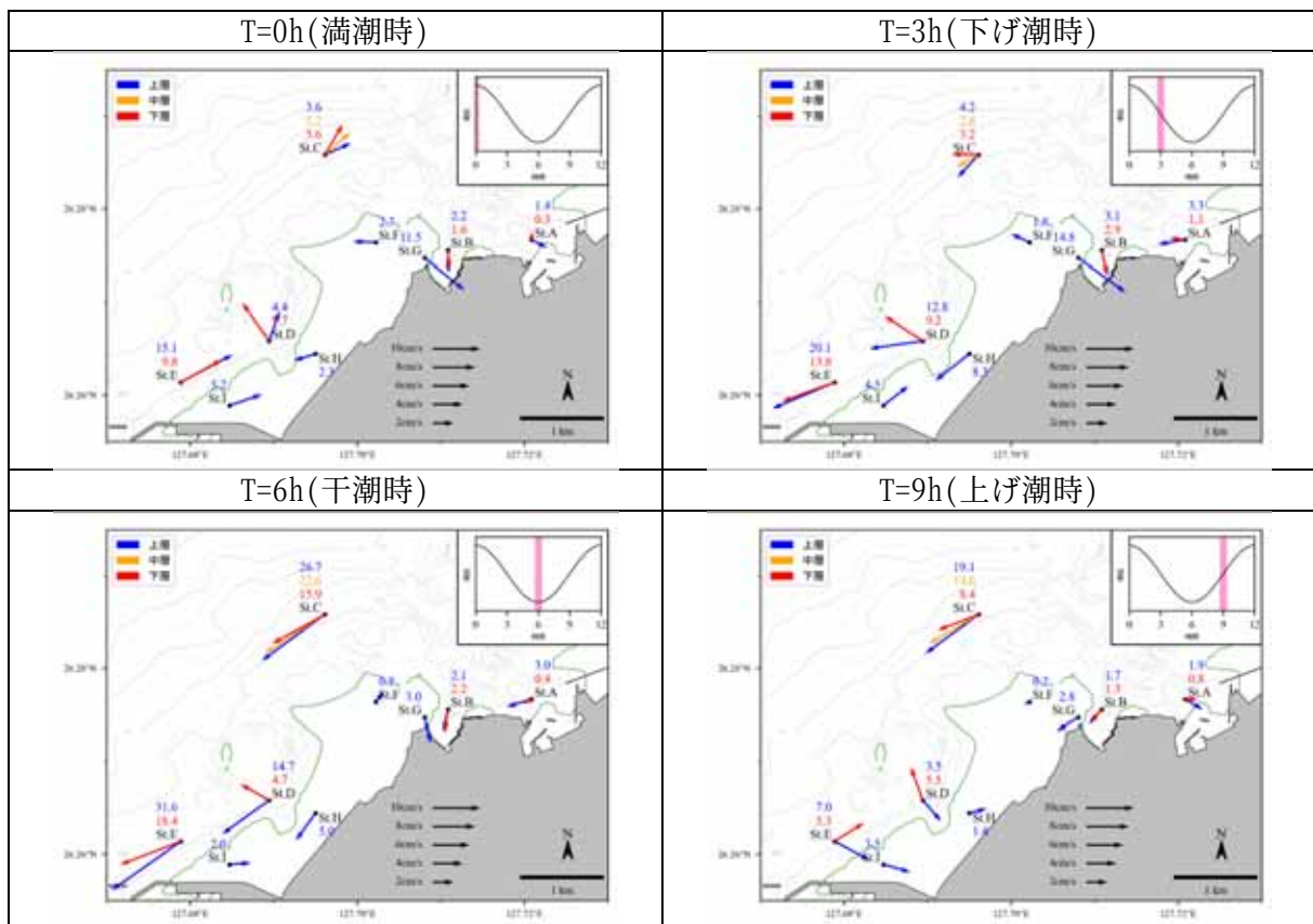
図 6.5.1.14 平均大潮期流況 (冬季)
