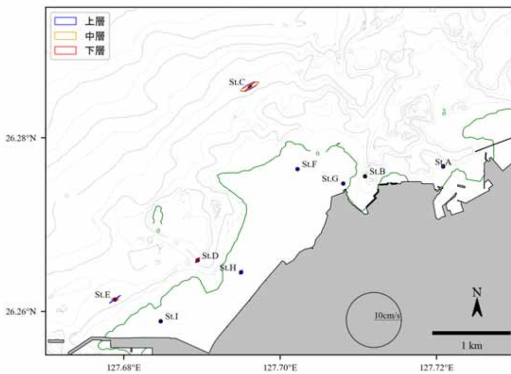
図 6.5.1.11(4) 主要 4 分潮の潮流橢円の平面分布図 ( O_1 分潮、夏季)
