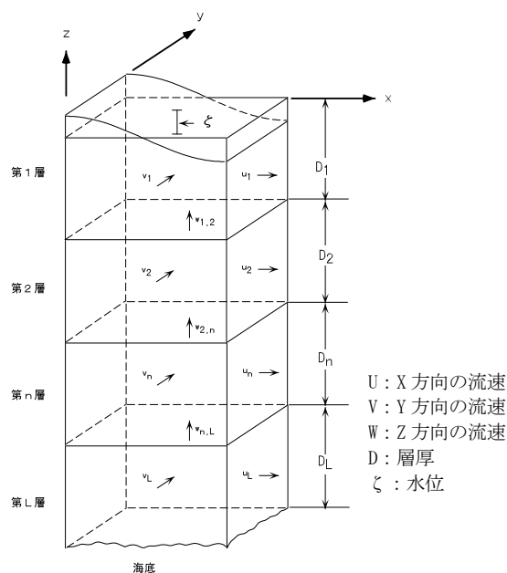
図 6.5.2.27 多層レベルモデルの概念図及び変数の定義点位置
