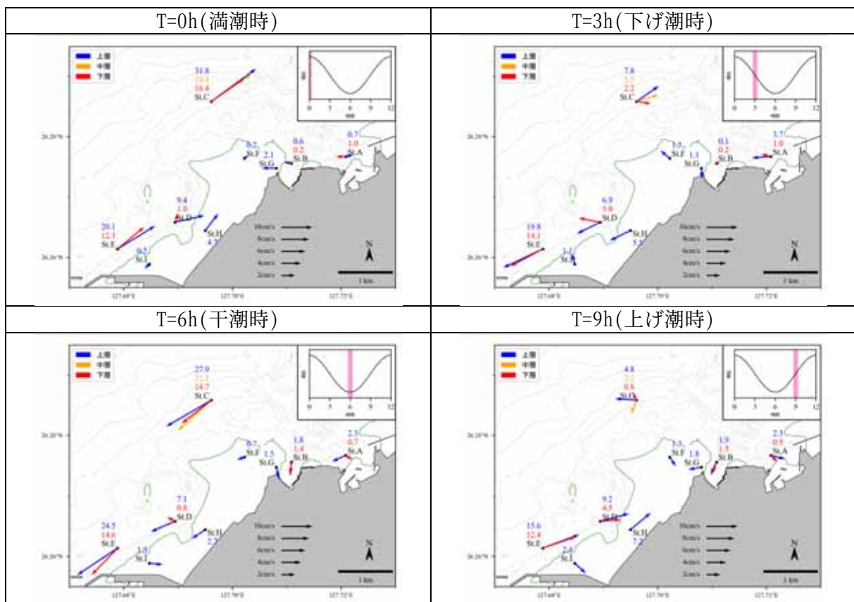
図 6.5.1.13 平均大潮期流況 (夏季)
