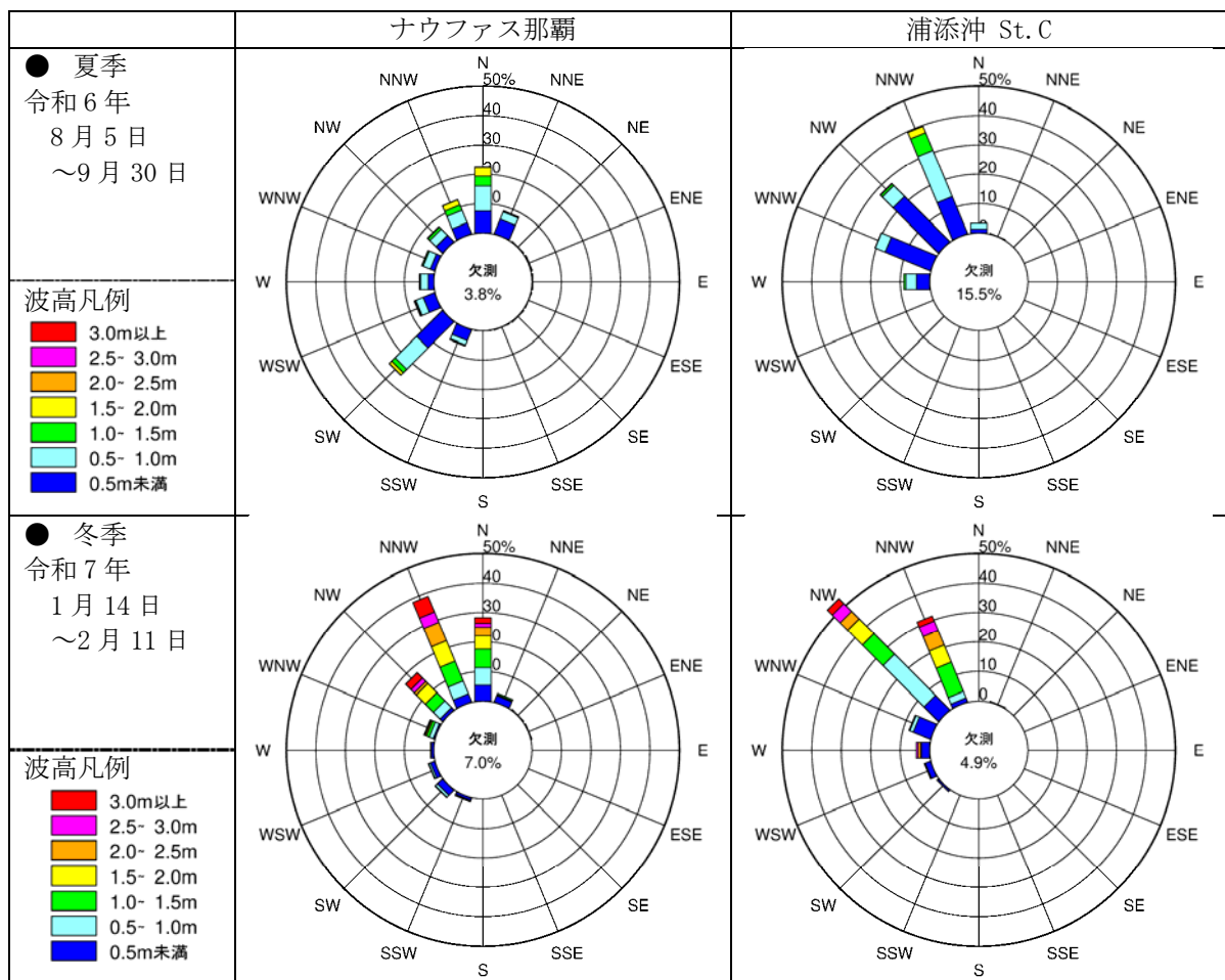
図 6.5.2.6 ナウファス那覇及び浦添沖 St. C の波高と波向の出現状況
