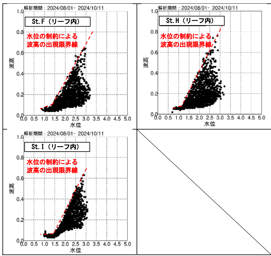
図 6.5.2.10 リーフ内 (St.F, H, I) の各地点における水位と波高の関係（全観測期間）
