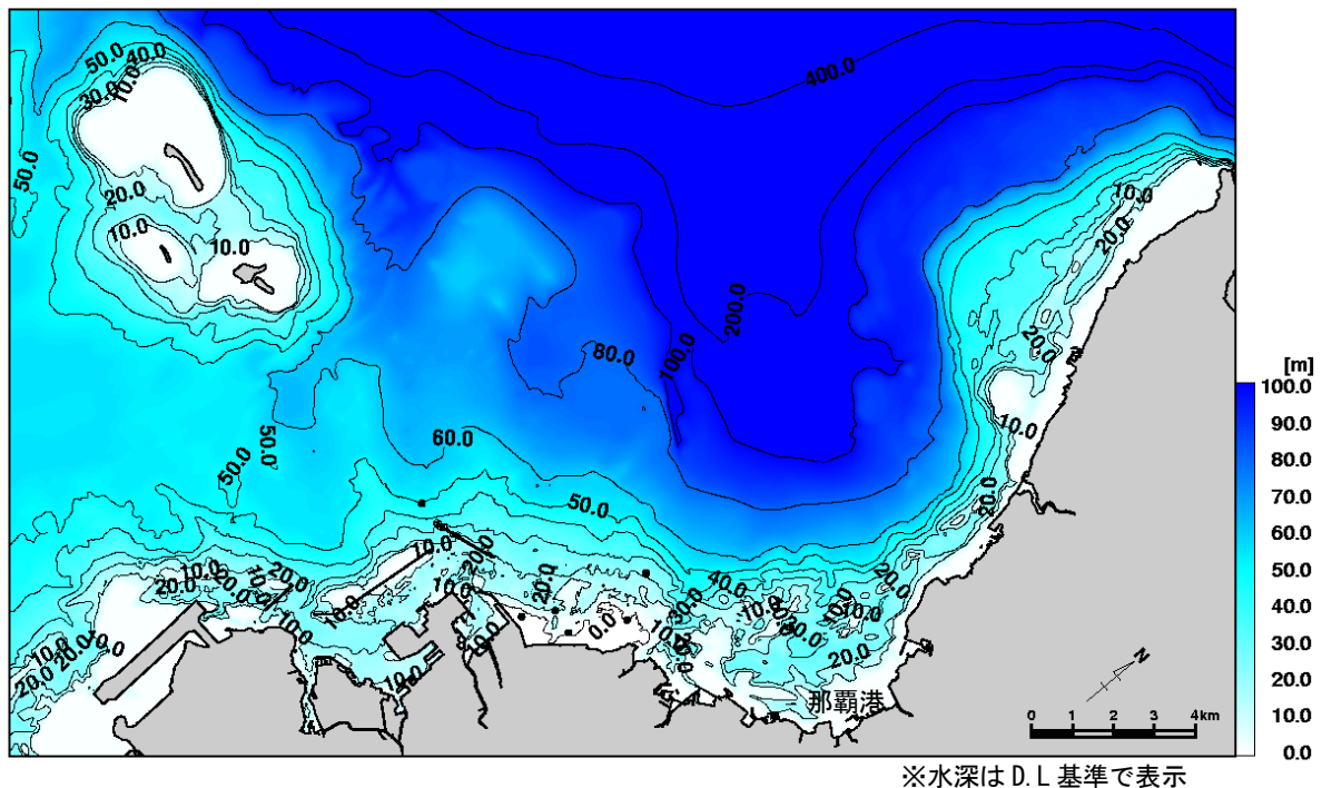
図 6.5.2.5 計算領域の水深図
