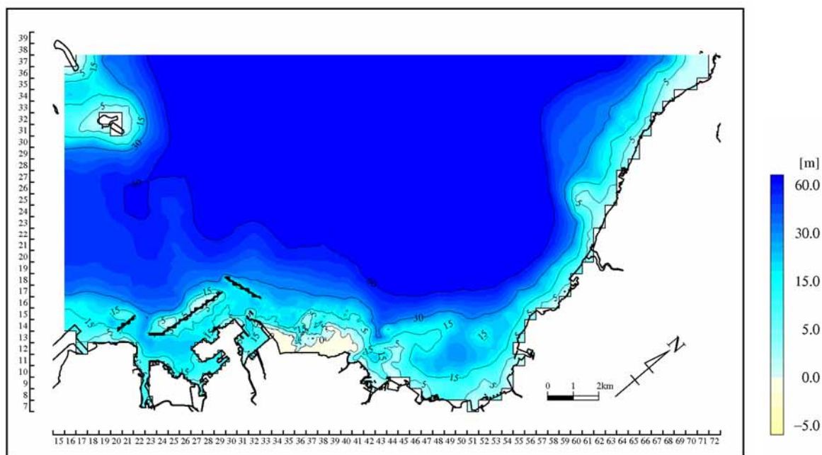
図 6.5.2.25(1) 計算範囲とその水深（単位：m DL 基準、緩衝領域：450m 格子）
