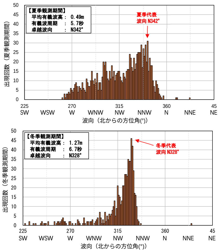
図 6.5.2.22 浦添沖(St. C)における季節別の波向出現状況
